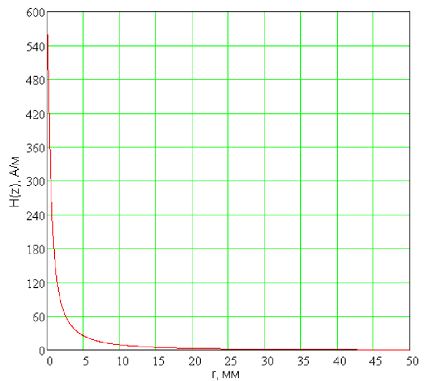
Рис. 3. Результаты моделирования зависимости напряженности магнитного поля H_{\Pi} созданного КПМ от расстояния r , отсчитываемого от боковой поверхности ПМ в горизонтальной плоскости, проходящей через его центр
