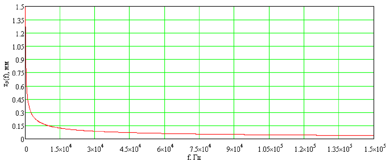
Рис. 2. Зависимость толщины эффективно проводящего z_3 -слоя в мм от частоты токовых импульсов в Гц для цилиндрического ВЛ при \gamma=1,15 \cdot 10^7 См/м, \mu_a=1,25 \cdot 10^{-4}
