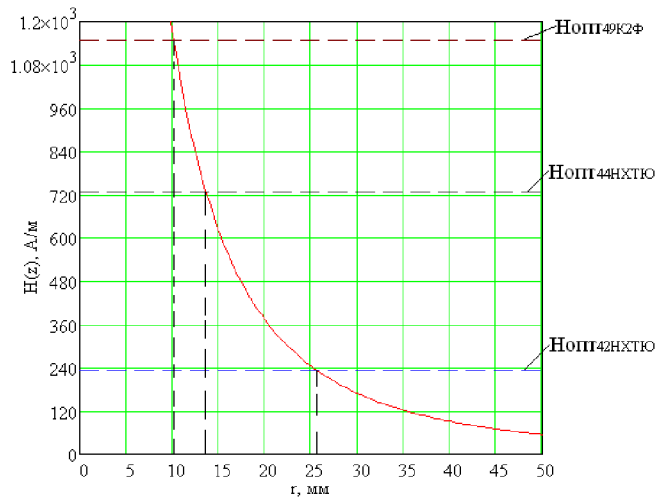
Рисунок 3. Результати дослідження в МУ с ППМ значень r_{MIN} , r_{OPT} і r_{MAX} при зміні марки ВЛ
