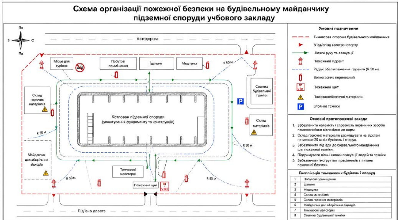
Рис. 1. Схема організації пожежної безпеки на будівельному майданчику
