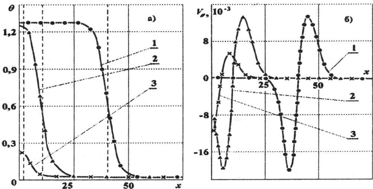
Рис. 1. Розподіл температури (а) та швидкості зміни температури (б) за товщиною двохшарової системи «частка зі сплаву Fe 83 B 17 — сталева основа» при Fo = 8,69 \cdot 10^{-12} , \theta_{10} = 1,28 для різних значень \delta_1 : 1 — \delta_1 = 40,0 ; 2 — 10,0 ; 3 — 1,0
