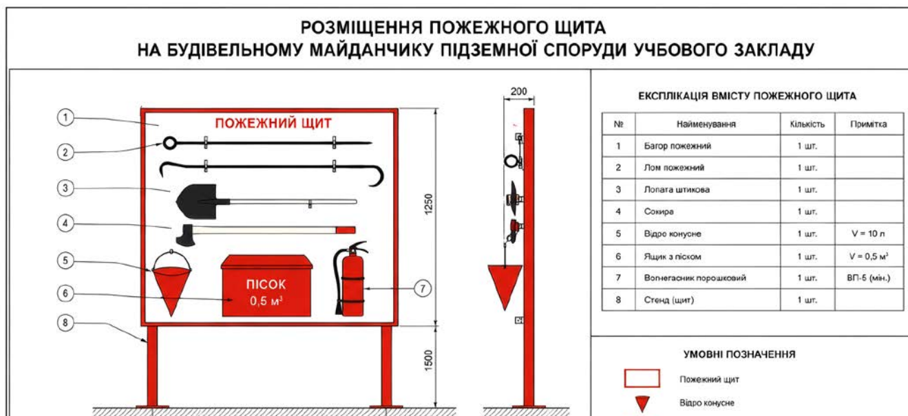
Рис. 2. Комплектація та розміщення пожежного щита Джерело: розробка авторів
