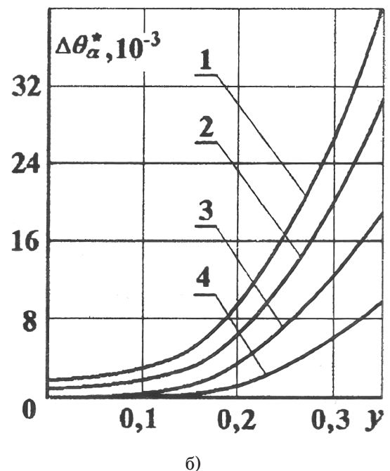
Рис. 2. Залежність \Delta\theta_\alpha^* = f(y) в системі «одношарове покриття-підшар-основа» для z = -3,075 за умов спеціального охолодження водою ( Bi_{y_0} = 1,49 ) вільної поверхні основи: 1 — x = 0 ; 2 — x = 0,53 ; 3 — x = 0,85 ; 4 — x = 1,12 ; а) при \Delta_1 = 0,34 ; б) при \Delta_1 = 0,17
