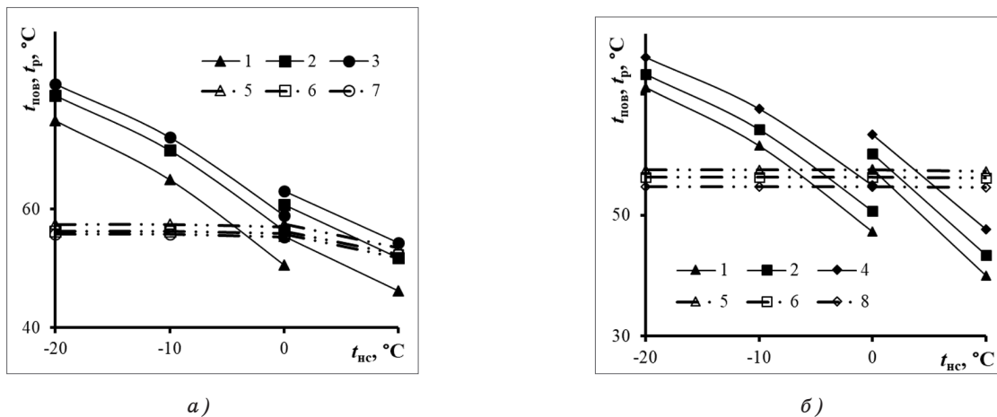
Рис. 3. Залежність температури внутрішньої поверхні t_{пов} у гирлі димової труби (1–4) і точки роси t_p (5–8) від температури навколишнього середовища t_{нс} при застосуванні повітряного методу для різних значень частки підмішуваного повітря \sigma та температури t_{zn} при температурі підмішуваного повітря t_{zn} = 150\text{ }^{\circ}\text{C} : 1, 5 — \sigma = 0\% ; 2, 6 — 8\% ; 3, 7 — 12\% ; 4, 8 — 20\% ; а) цегляна димова труба при t_{zn} = 160\text{ }^{\circ}\text{C} ; б) металева димова труба при t_{zn} = 200\text{ }^{\circ}\text{C}
