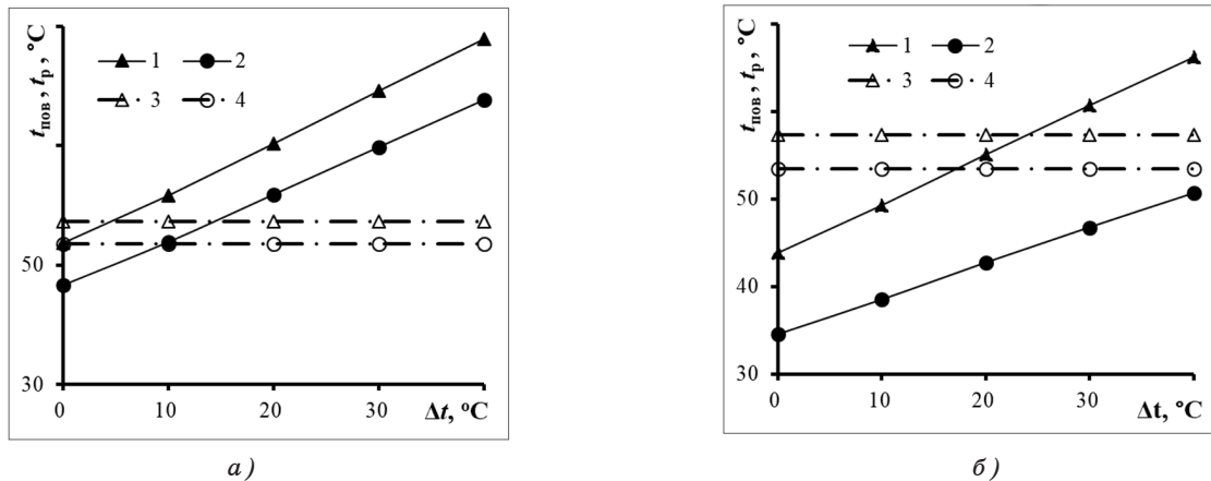
Рис. 2. Залежність температури внутрішньої поверхні t_{пов} у гирлі димової труби (1–2) і точки роси t_p (3–4) від величини \Delta t при температурі навколишнього середовища t_{нс} = 10\text{ }^{\circ}\text{C} для різних значень температури t_{zn} : 1, 3 — t_{zn} = 200\text{ }^{\circ}\text{C} ; 2, 4 — 160\text{ }^{\circ}\text{C} ; а) цегляна димова труба; б) металева димова труба.
