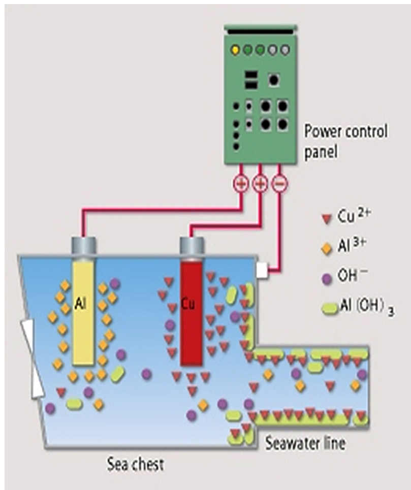
Рис. 1. Система MGPS кінгстонного типу (MGPS SEA CHEST TYPE)
