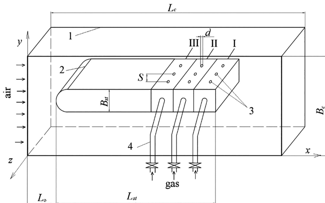
Рис. 1. Схема модуля мікрофакельного пальника стабілізаторного типу з трирядною системою подачі палива:
