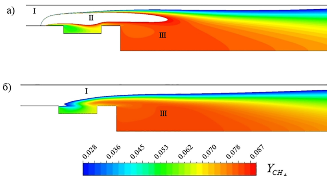
Рис. 4. Поля масової концентрації метану в поздовжньому перерізі циліндричного стабілізаторного паливника потужністю 110 кВт, що проходить через центр газоподавального отвору (а) та посередині між отворами (б)
