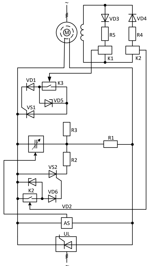
Рис. 1. Принципова схема керування при циклічному керуванні параметрами контуру збудження СД з ЄНЕ
