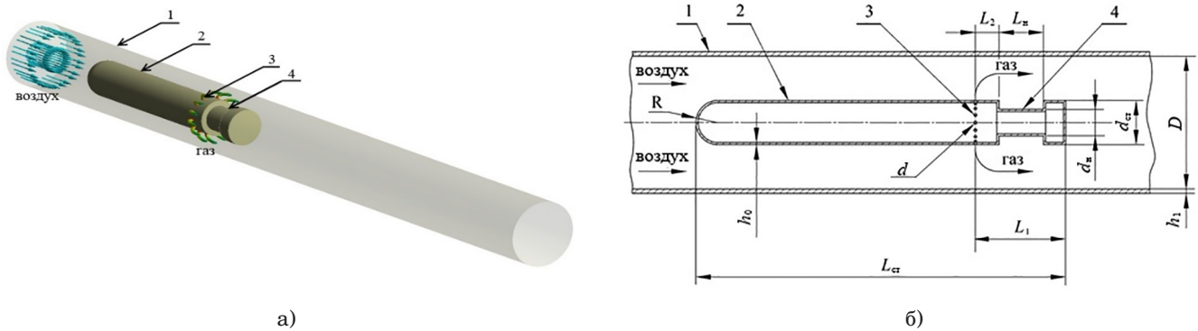
Рис. 1. Схема (а) та поздовжній переріз (б) пальникового пристрою з циліндричним стабілізатором полум'я: 1 — круглий канал; 2 — циліндричний стабілізатор полум'я; 3 — газоподавальні отвори; 4 — кільцева ніша
