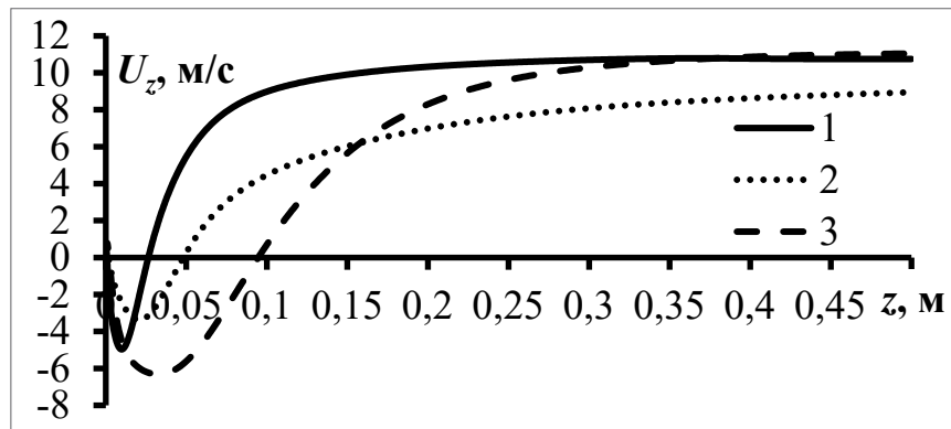
Рис. 3. Розподіл осевої компоненти швидкості U_z вздовж осі турбулентного сліду за циліндричним стабілізатором полум'я для паликових пристроїв різної потужності N_n : 1 — N_n = 20 кВт; 2 — N_n = 110 кВт; 3 — N_n = 200 кВт
