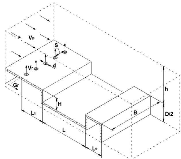
Рис. 2. До постановки задачі при використанні другої (уточненої) моделі витікання палива через газоподавальні отвори
