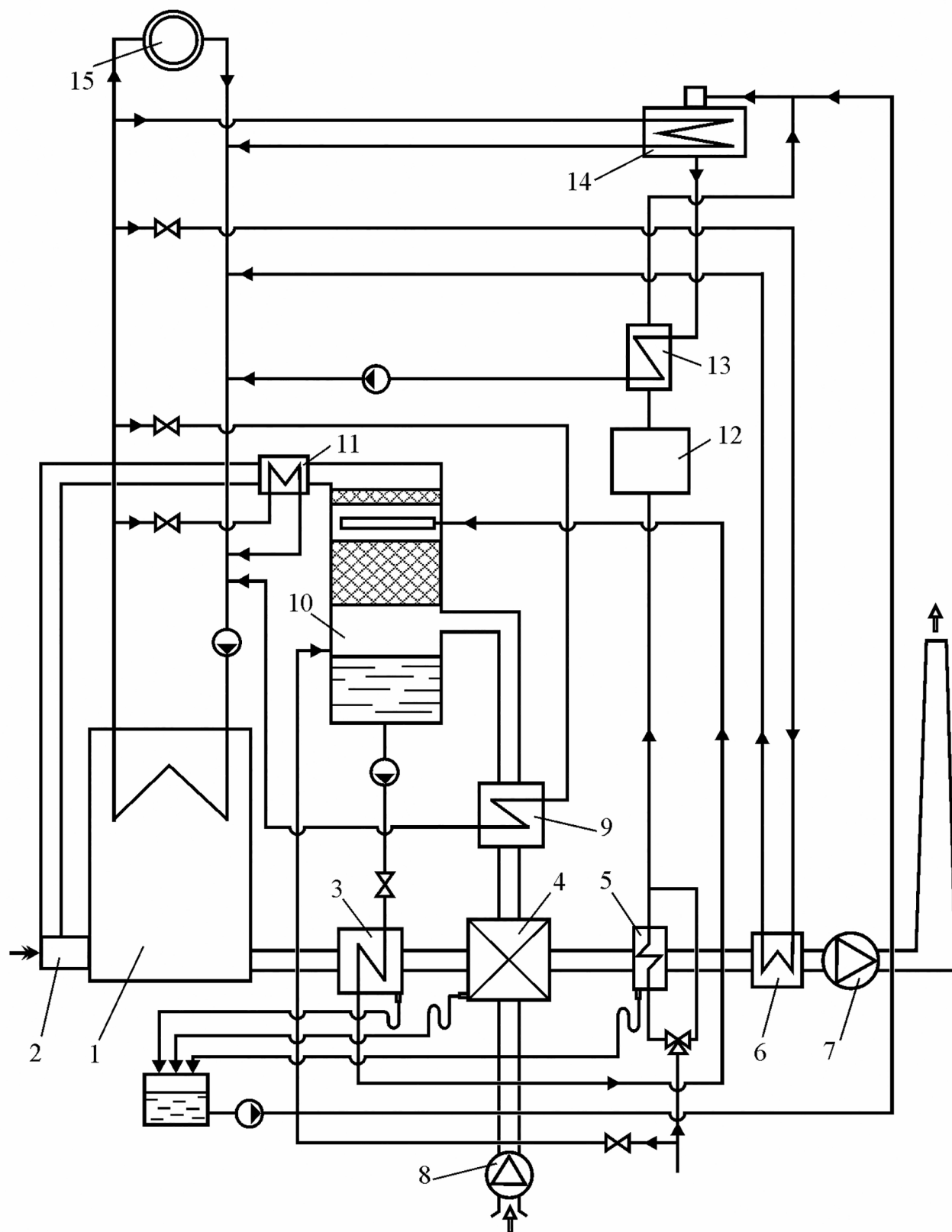
Рис. 1. Котельня установка з комбінованим використанням утилізованої теплоти: 1 — котлоагрегат; 2 — газопальниковий пристрій; 3 — водопідігрівач; 4 — повітропідігрівач; 5 — підігрівач холодної води на ХВО; 6 — газопідігрівач; 7 — димосос; 8 — вентилятор; 9 — водоповітряний теплообмінник; 10 — контактний водоповітряний тепломасообмінник; 11 — повітродогрівач; 12 — система ХВО; 13 — підігрівач хімічно очищеної води; 14 — деаератор; 15 — споживач
