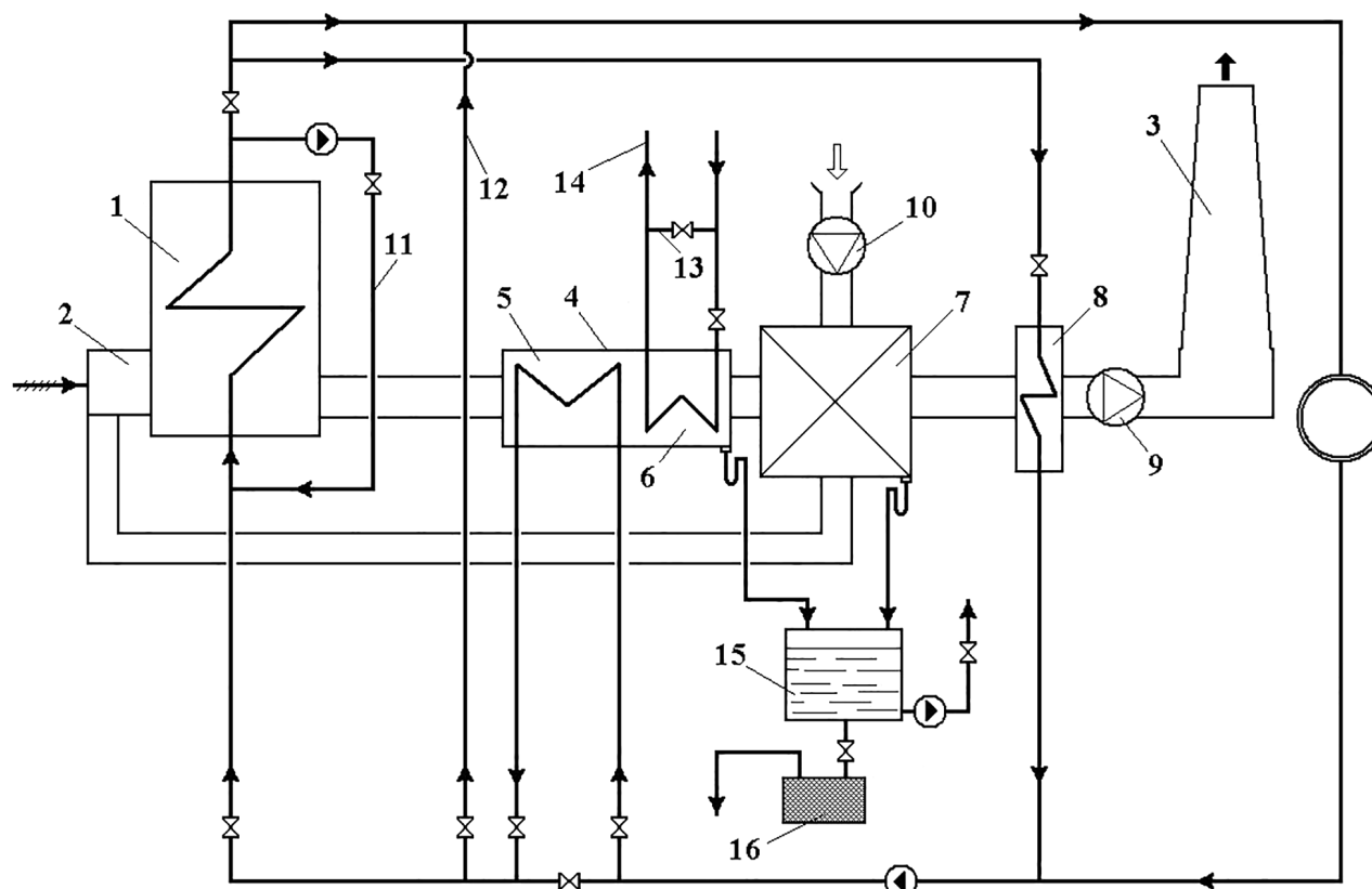
Рис. 1. Котельня установка з комбінованим використанням утилізованої теплоти:
