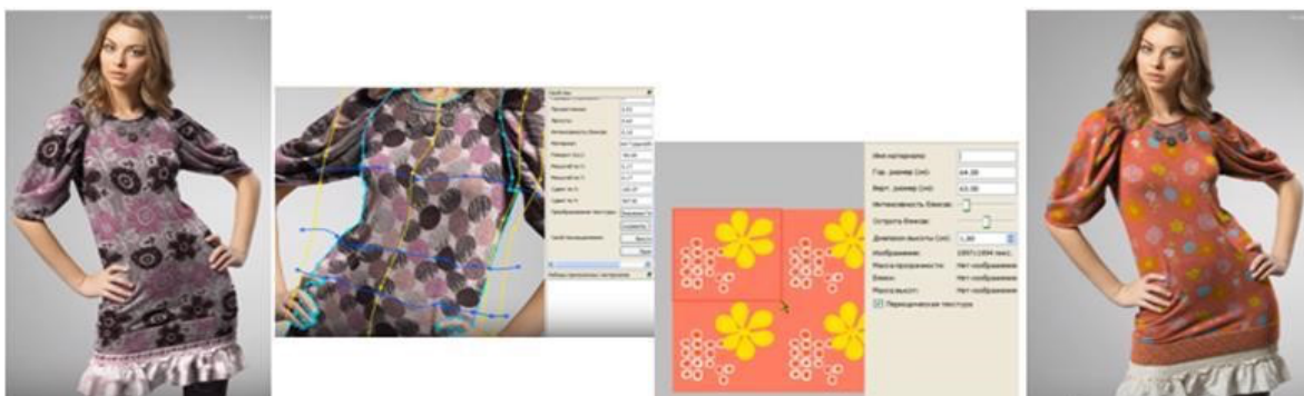
Рис. 8. Візуалізація форми виробу в двовимірному модулі Assyst [10]
