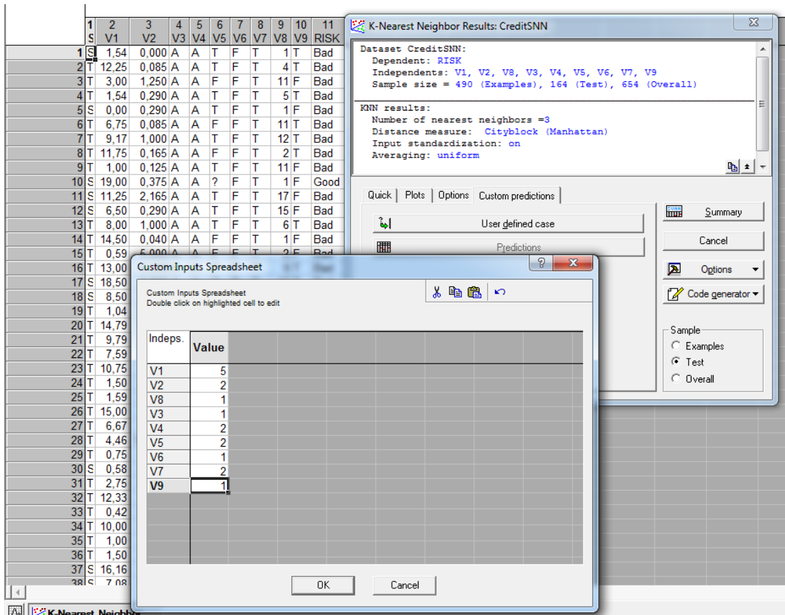
Рис. 1. Приклад конфігурованої автором та тренованої kNN моделі машинного навчання для бінарної класифікації ризикованості нових контрагентів компанії зі сфери готельно-ресторанного бізнесу. (використаний набір даних CreditSNN, автором визначені такі оптимальні параметри моделі: k=3 , міра відстані = Манхеттенівська, в якості попередньої обробки даних виконана стандартизація значень, налаштування усереднення відповіді (з по між 3х відібраних аналогічних випадків дата сету) = uniform
