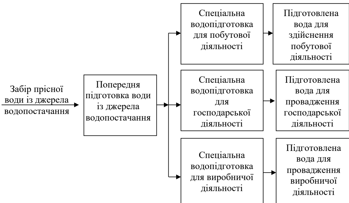
Рис. 3. Укрупнена структура підготовки прісної води
