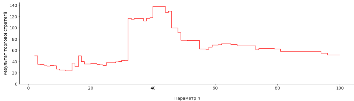
Рис. 9. Результати ЕМА з 10.08.2022 по 05.07.2024 без врахування комісійних
