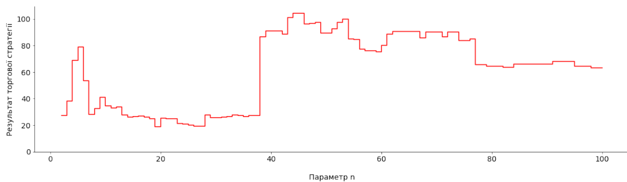
Рис. 11. Результати LWMA з 10.08.2022 по 05.07.2024 без врахування комісійних
