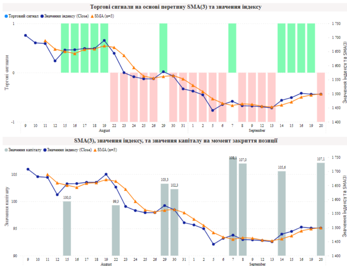
Рис. 5. Значення індексу та плинної середньої разом із розрахованими торговими сигналами та зміною капіталу
