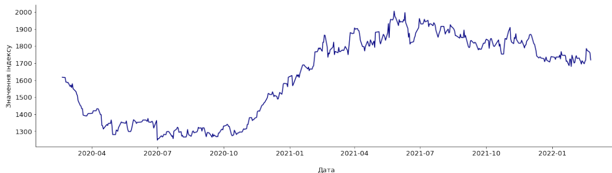
Рис. 4. Динаміка індексу UX за період з 20.02.2020 по 23.02.2022
