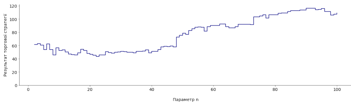
Рис. 10. Результати ЕМА з 20.02.2020 по 23.02.2022 без врахування комісійних
