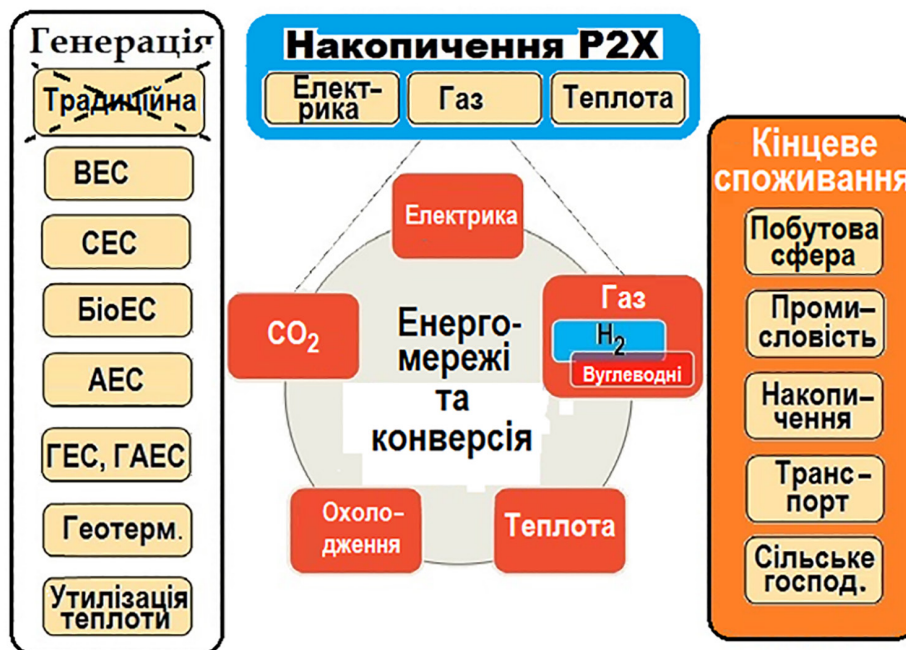
Рис. 1. Галузеве сполучення в інтегрованих системах енергопостачання/енергоспоживання за концепцією P2X (Power-to-X; {X}=(H=Heat, G=Gas= \text{H}_2 / \text{CH}_4 )). (ВЕС — вітряна енергетична станція, СЕС — сонячна електростанція, БіоЕС — електростанція на біопаливі, АЕС — атомна електростанція, ГЕС — гідроелектростанція, ГАЕС-гідроакumuлююча електростанція) [4]
