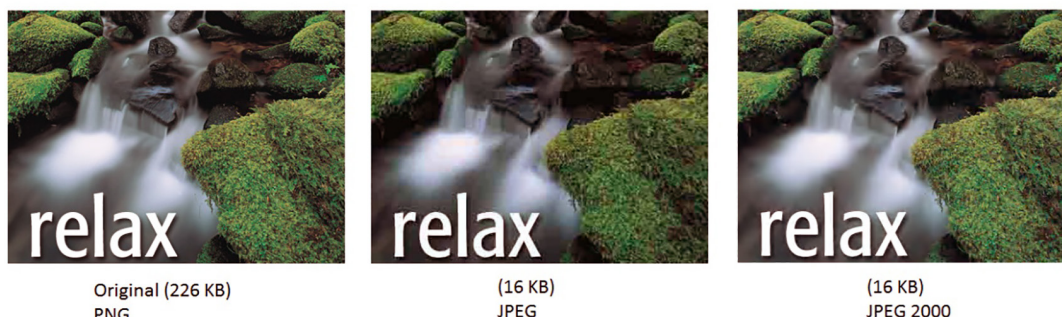
Рис. 2. Порівняння алгоритмів
