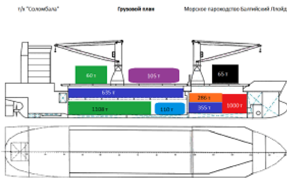
Рис. 1. Попередні одно та двохплощинні вантажні плани
