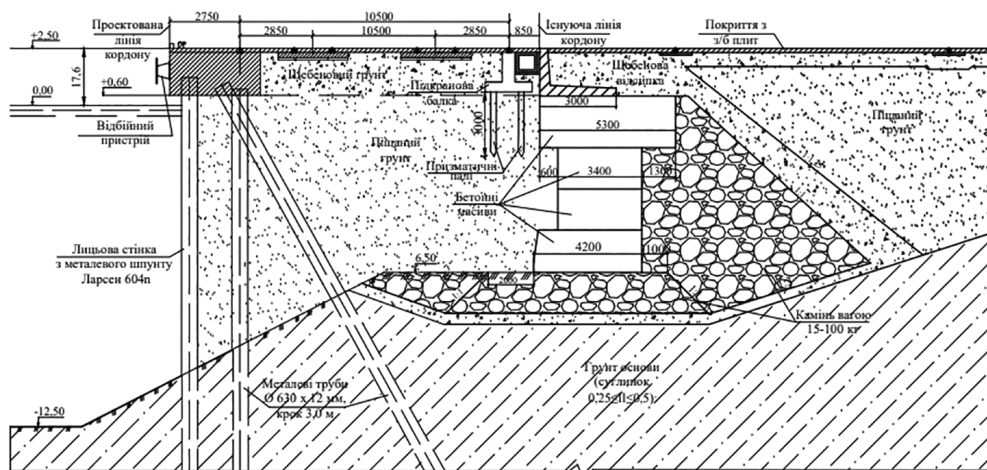
Рис. 2. Схема причалу після реконструкції
