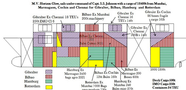
Рис. 1. Попередні одно та двохплощинні вантажні плани
