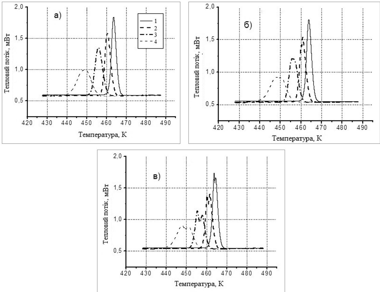
Рис. 1. Екзотерми кристалізації для полімерних композиційних матеріалів на основі полікарбонату, наповнених мікрочастинками алюмінію, при вмісті наповнювача \omega = 0,2\% (а), 1,0 (б) и 4,0\% (в)
