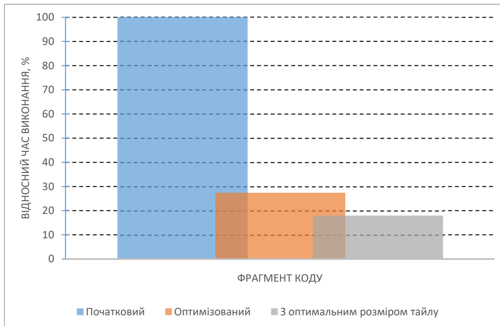
Рис. 6. Порівняння часу виконання оптимізованих фрагментів коду з розміром тайлу за замовчуванням та оптимальним
