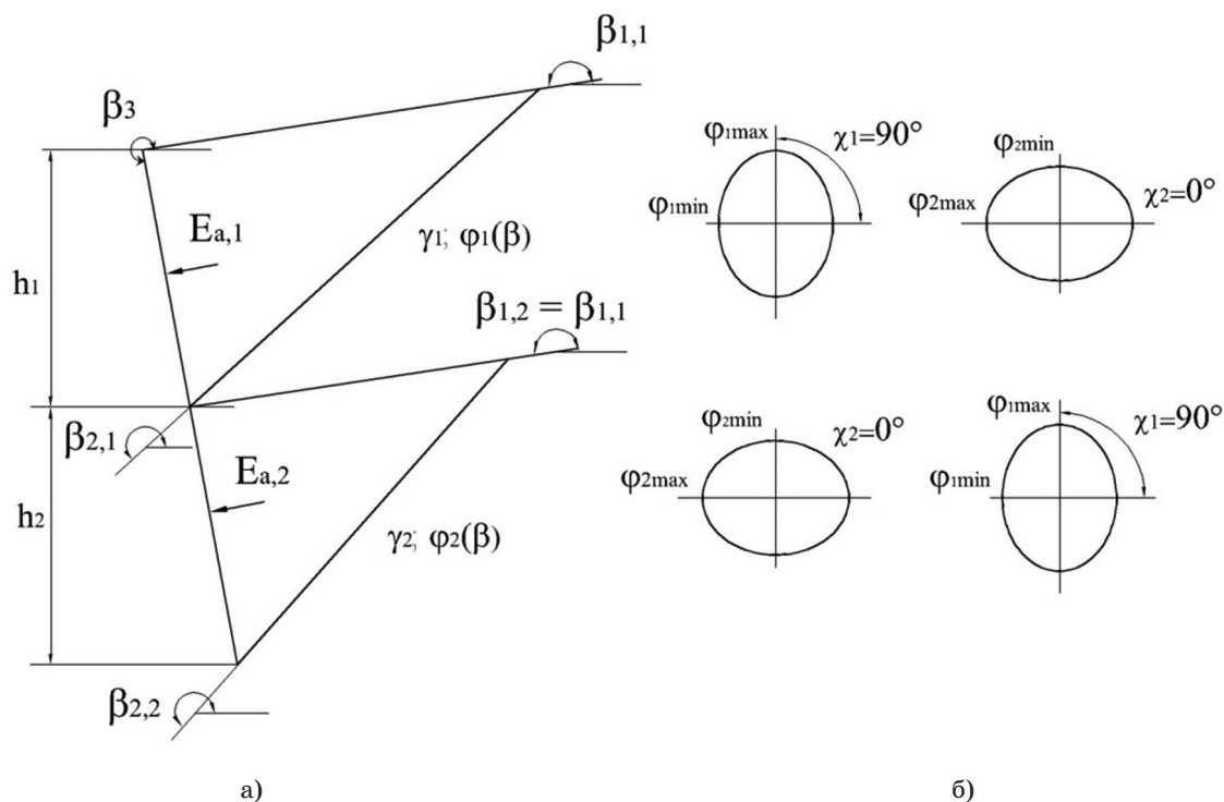
Рис. 2. Розрахункова схема (а) і варіанти комбінацій годографів кута внутрішнього тертя \varphi ( \beta ) при орієнтації вісі максимальної міцності n -го шару ґрунту \chi_n (б)
