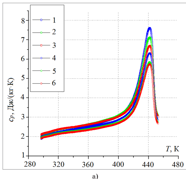
Рис 1. Залежність теплоємності наноконполитів від температури T для різних значень масової частки наповнювача \omega та часу змішування \tau :
