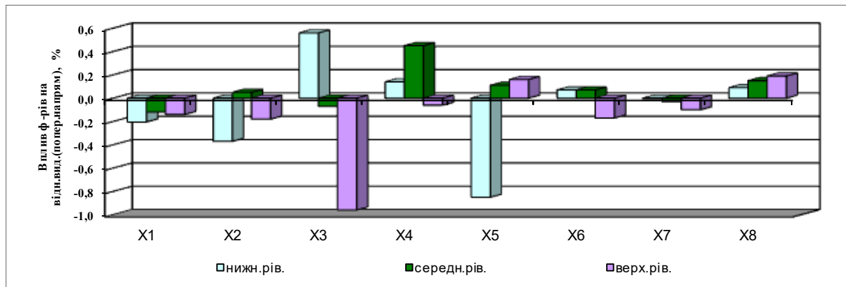
Рис. 4. Вплив вхідних факторів паперу-основи та компонентів складу на показник відносного видовження (у поперечному напрямку) ( Y_{\text{в.вид.}(п.н.)} )
