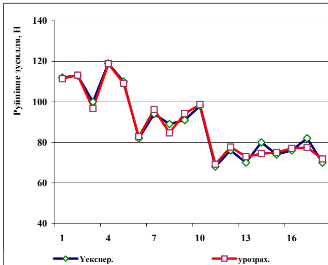
Рис. 1. Порівняльні характеристики моделі за параметром Y_{руйнів}
