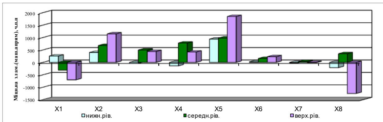
Рис. 5. Вплив вхідних факторів паперу-основи та компонентів складу на показник міцності на злом (у машинному напрямку) ( Y_{\text{злом.}(м.н.)} )
