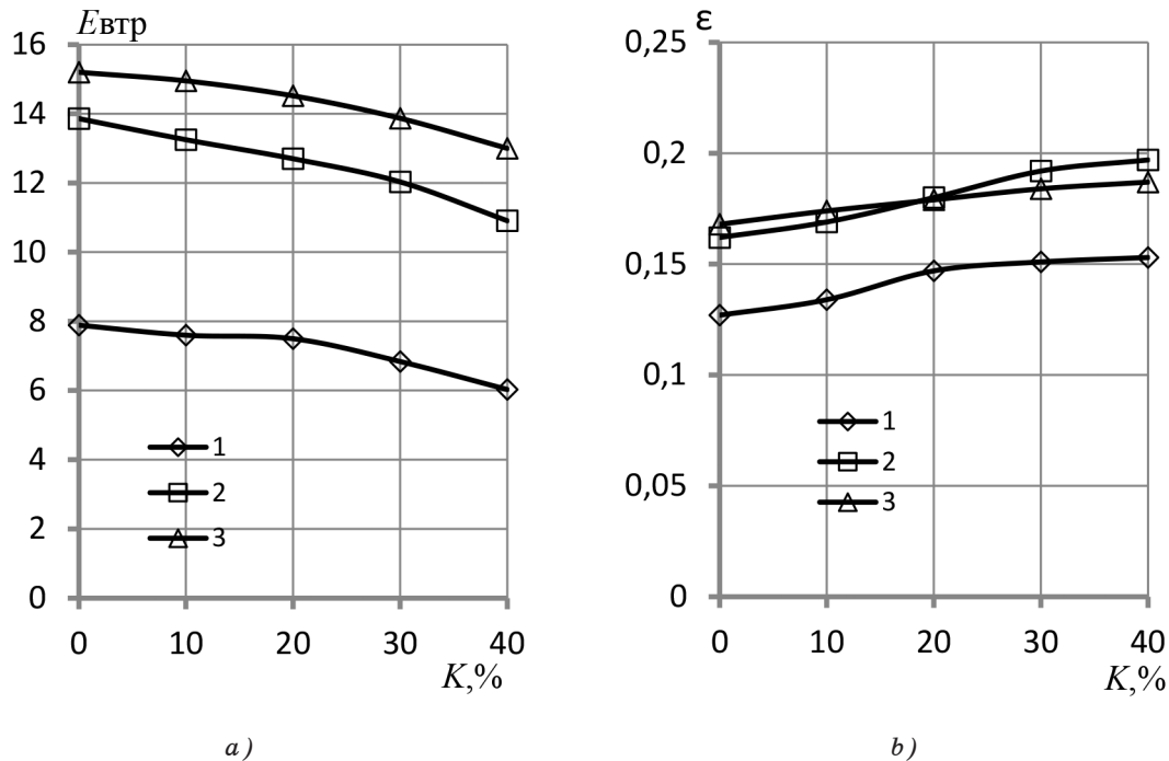
Рис. 2. Залежність ексергетичних втрат E_{\text{ex}} та тепло-ексергетичного критерія ефективності \varepsilon від кількості байпасованих димових газів K для методу байпасування: 1 — Q = 62,3\text{--}39,5\text{ кВт} ; 2 — 85,5\text{--}55,4\text{ кВт} ; 3 — 90,7\text{--}69,5\text{ кВт}
