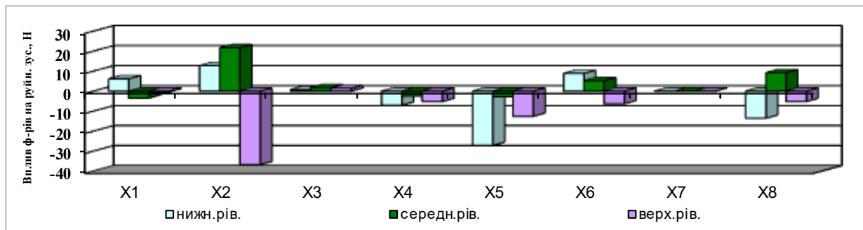
Рис. 2. Вплив вхідних досліджуваних факторів паперу-основи та компонентів складу на показник руйнівного зусилля ( Y_{руйнів.} )
