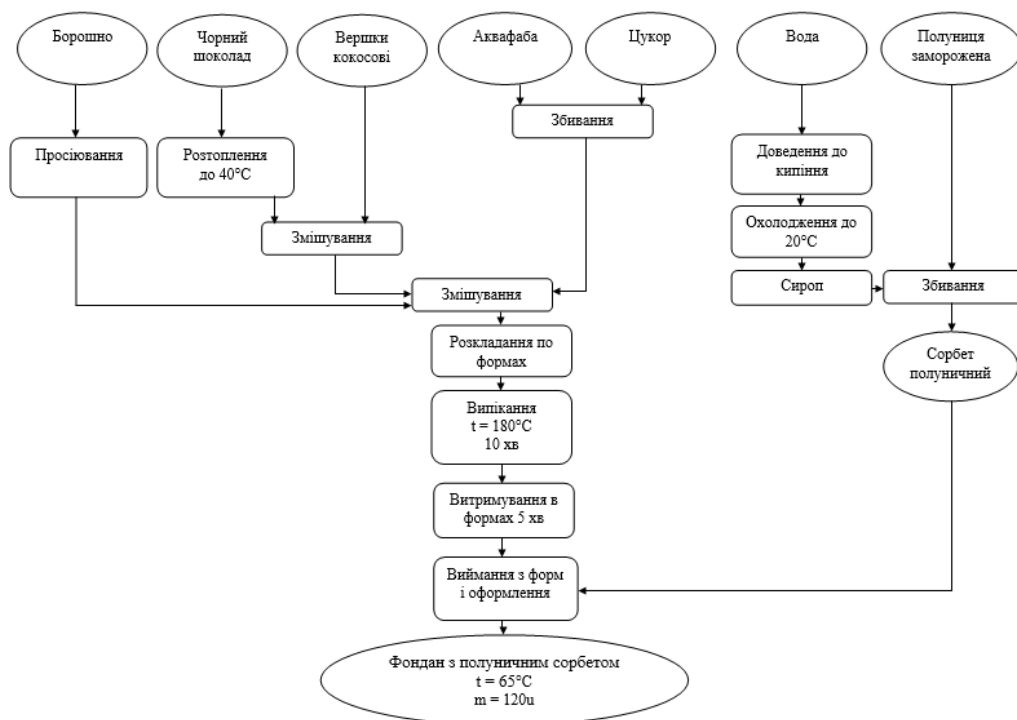
Рис. 3. Параметро-технологічна схема фондану з полунциним сорбетом
