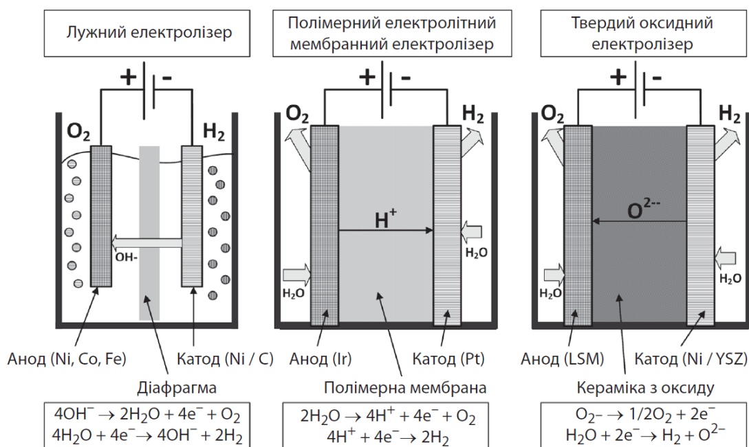
Рис. 1. Принципи здійснення лужного, PEM і SOE електролізу [13; 14]
