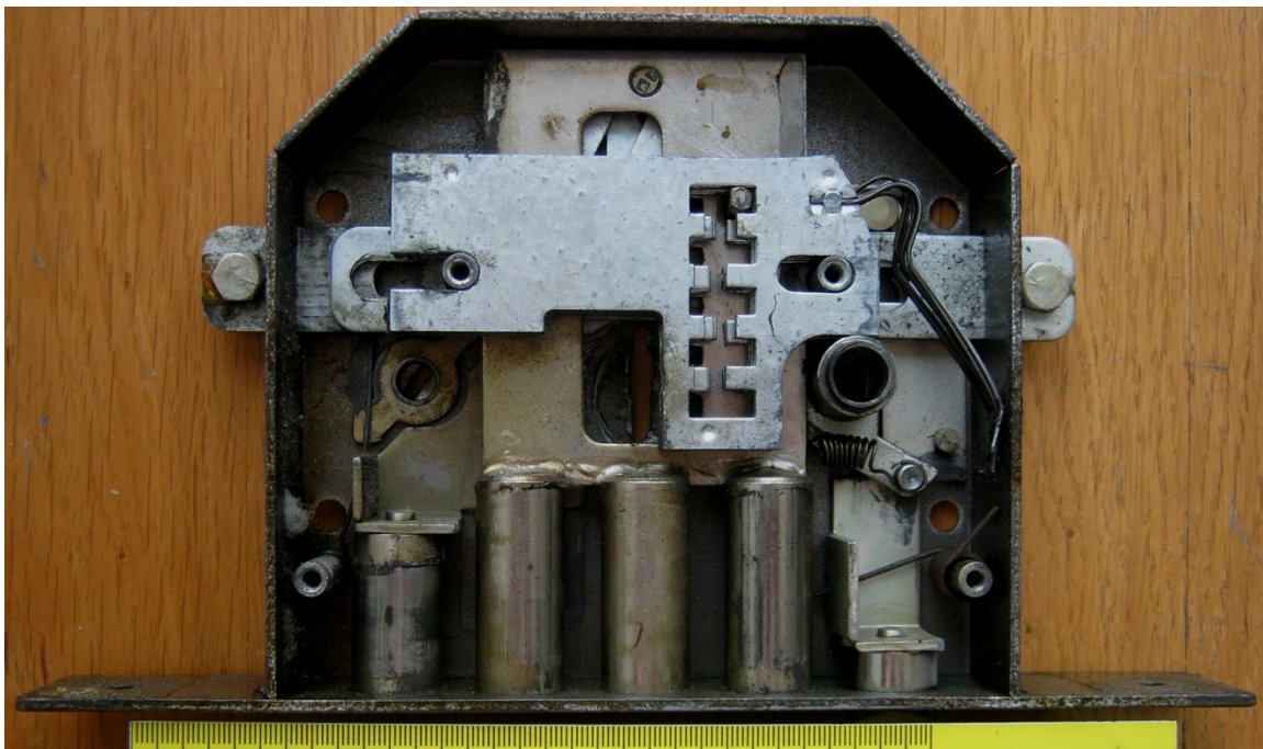
Рис. 4. Деталі сувальдного механізму замку, наданого на дослідження
