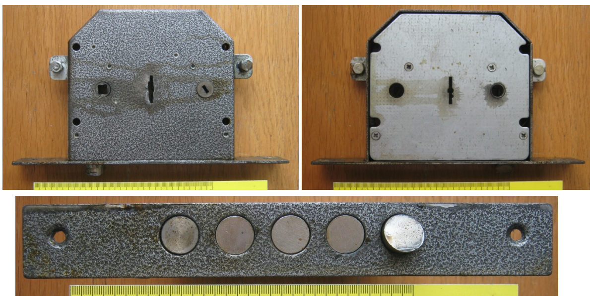
Рис. 1-3. Замок с сувальдним механізмом замикання, наданий на дослідження
