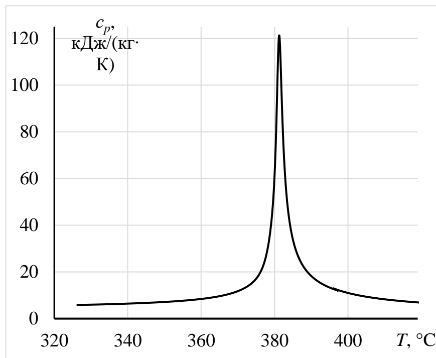
Рис. 3. Зависимость от температуры удельной теплоемкости сверхкритической воды при P = 24 МПа
