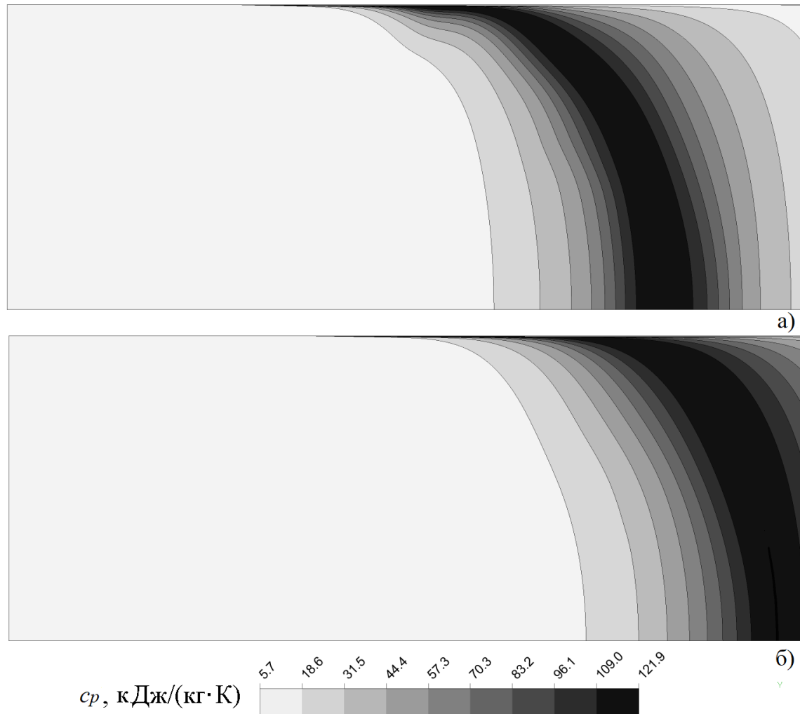
Рис. 1. Поля удельной теплоемкости c_p сверхкритической воды в канале при разных значениях подводимого к стенке теплового потока:
