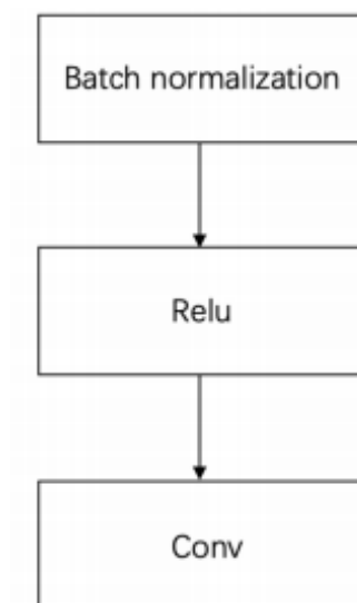
Рис. 3. Блок згортки
