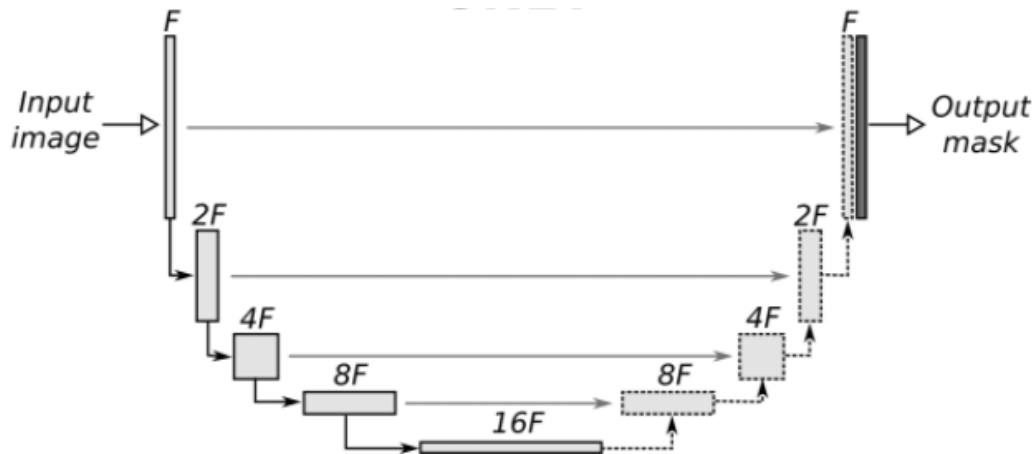
Рис. 2. Архітектура UNet
