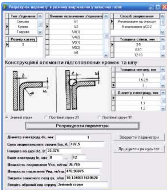
Рис. 3. Параметри зварювання у захисних газах: а) розрахунок; б) перевірка
