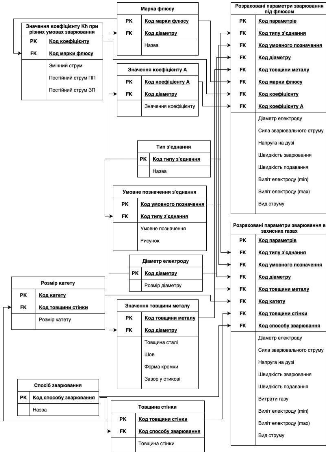
Рис.1. Логічна структура таблиць бази даних
