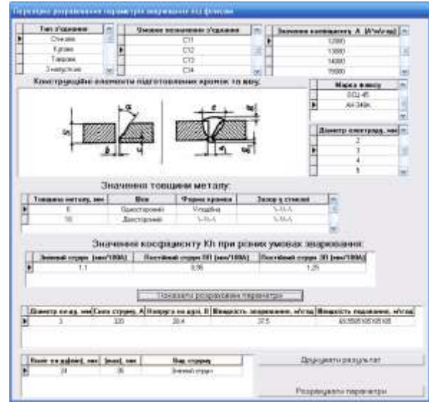
Рис. 2. Параметри зварювання під флюсом: а) розрахунок; б) перевірка
