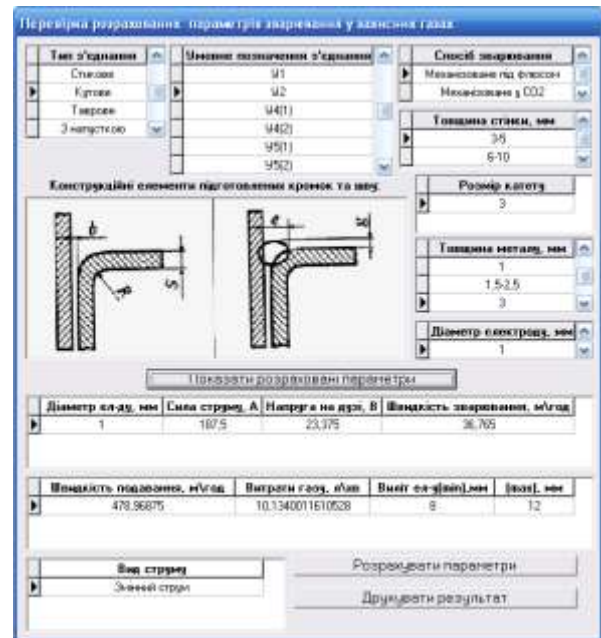
Рис. 3. Параметри зварювання у захисних газах: а) розрахунок; б) перевірка
