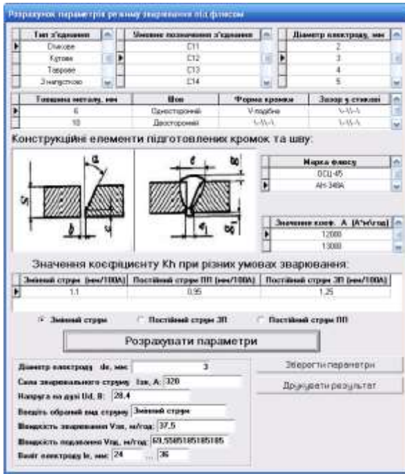
Рис. 2. Параметри зварювання під флюсом: а) розрахунок; б) перевірка
