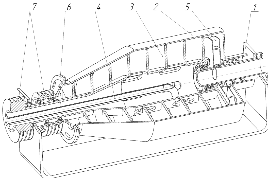
1 — корпус; 2 — ротор; 3 — шнек вивантаження осаду; 4 — штуцер завантаження суспензії; 5 — нерухоме робоче колесо з лопатями; 6 — отвори вивантаження осаду; 7 — шкві для приводу ротора та шнеку. Рис. 2. Модернізована конструкція осаджувальної центрифуги з пристроєм відводу фугату [5]
