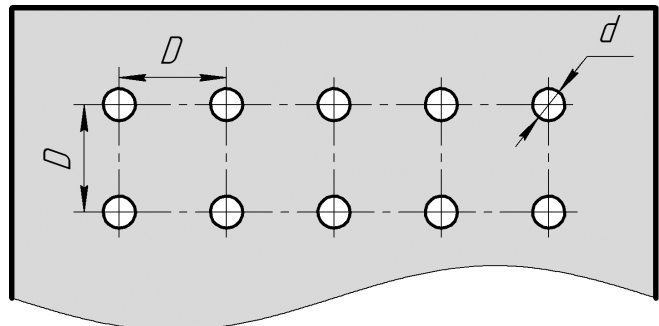
Рис. 6. Расположение отверстий в перфорированном экране
