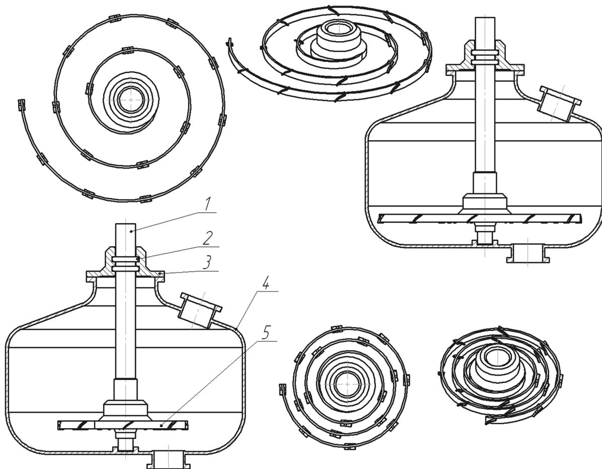
Рис. 1. Типова конструкція апарату з мішалкою, що містить гнучкі спіральні елементи
