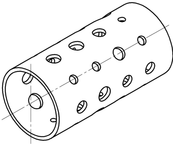
Рис. 5. Теплоизолирующий кожух с резонаторами
