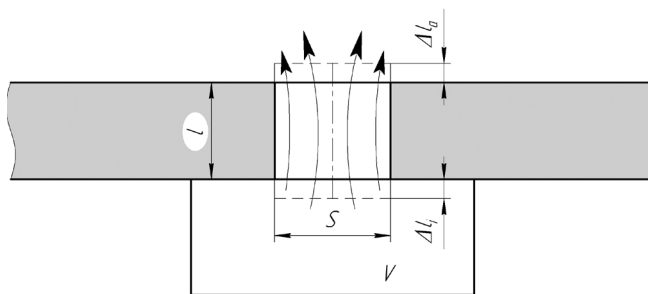
Рис. 1. Резонатор Гельмгольца
