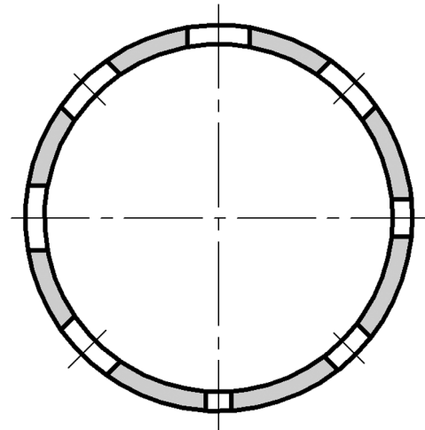
Рис. 5. Теплоизолирующий кожух с резонаторами
