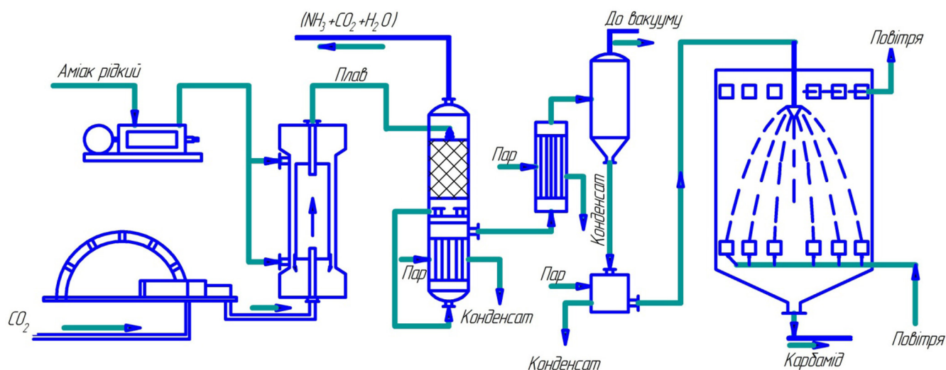
Рис. 1. Технологічна схема виробництва карбаміда
