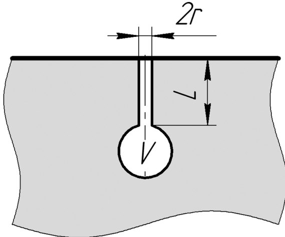
Рис. 7. Резонатор Гельмгольца
