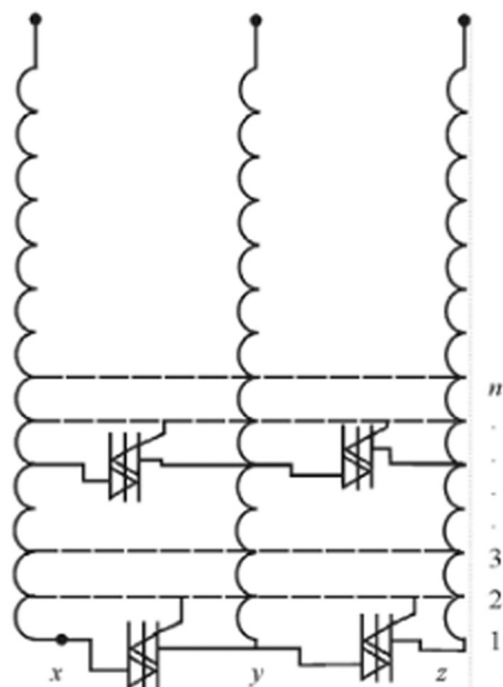
Рис. 2. Симісторний комутатор відгалужень трансформатора
