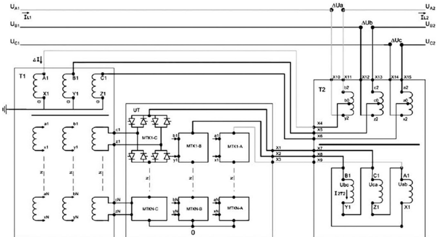
Рис. 3. Функціональна схема ФПТ з тиристорним комутатором
