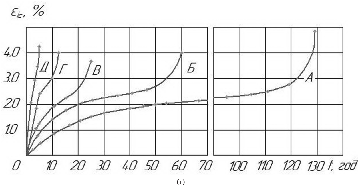
Рис. 2 в, г Криві повзучості сталі 15X2MΦA ( T = 550^\circ\text{C} ) при \varphi = -\pi/4 (в) і \varphi = \pi/2 (г):
