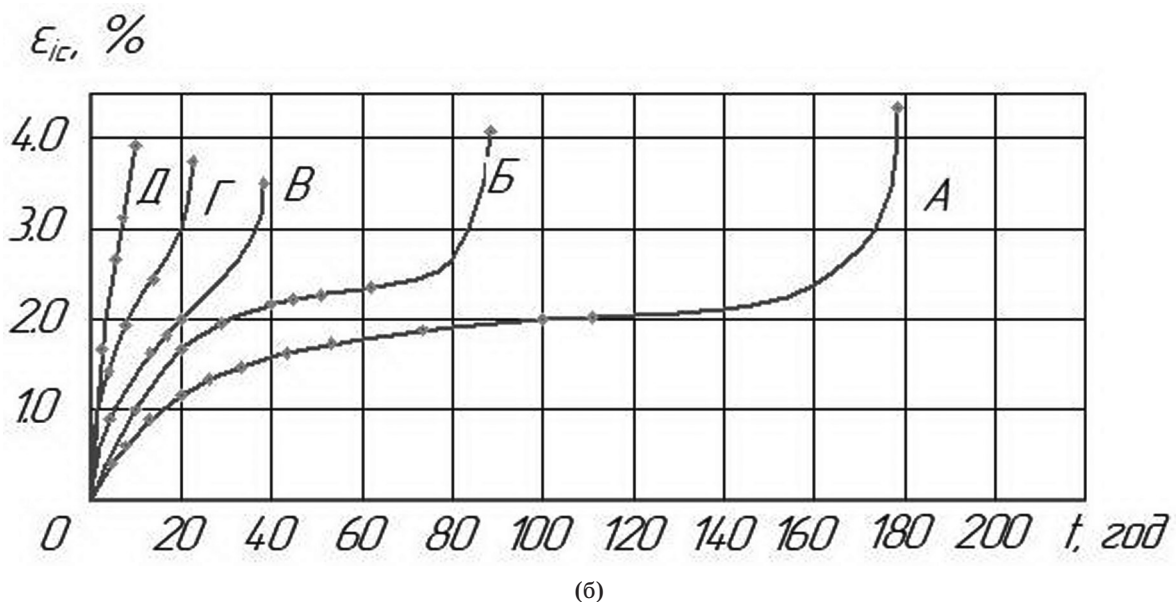
Рис. 2 а, б Криві повзучості сталі 15Х2МФА ( T=550^\circ\text{C} ) при \varphi=0 (а) і \varphi=\pi/3 (б):
