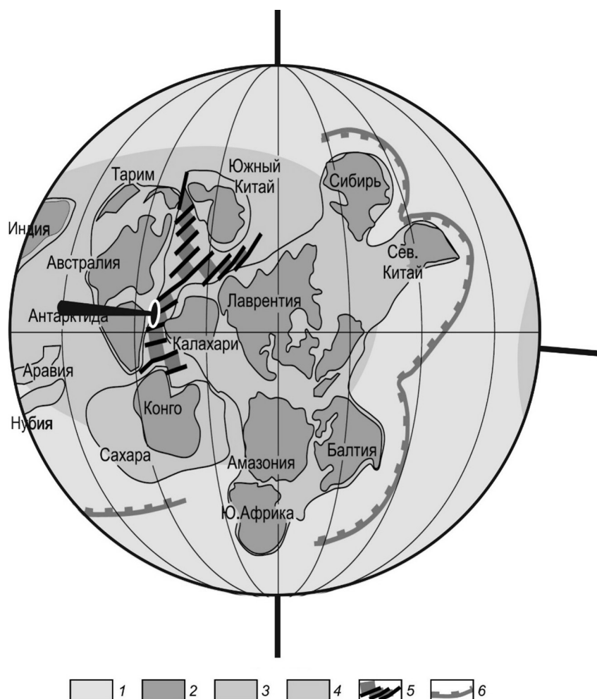
Рис. 2. Суперплюм, расколовший Родинию, и антиподальный суперплюм в океане.
