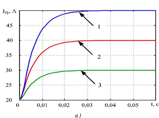
Рис. 3. Розрахункові залежності режимів форсування напруги збудження СГ: а) некомпенсованого контуру; б) компенсованого контуру
