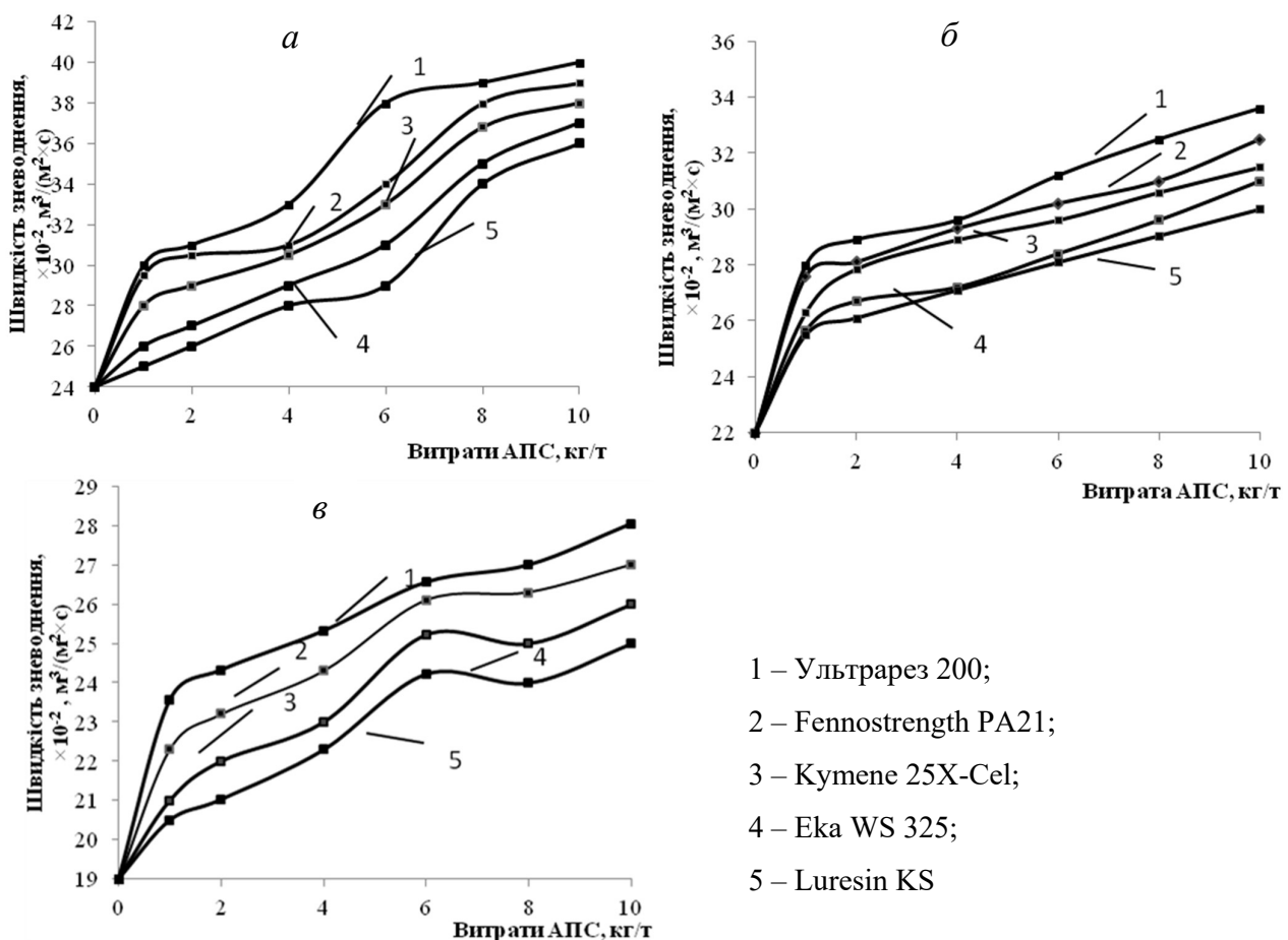
Рис. 3. Залежність швидкості зневоднення волокнистої маси із макулатури марки МС-5Б-2 від витрат АПС за температури 30^{\circ}\text{C} і ступеня млива 45^{\circ}\text{ШР} (а), 50^{\circ}\text{ШР} (б) і 55^{\circ}\text{ШР} (в)
