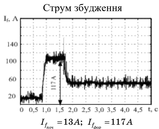
Рис. 5. Режим підключення АД до СГ з компенсованим контуром збудження
