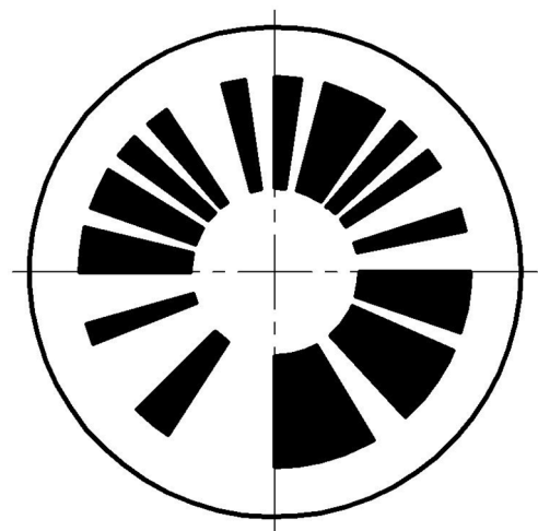
Рис. 6. Ротор пневматичної сирени: m=59
