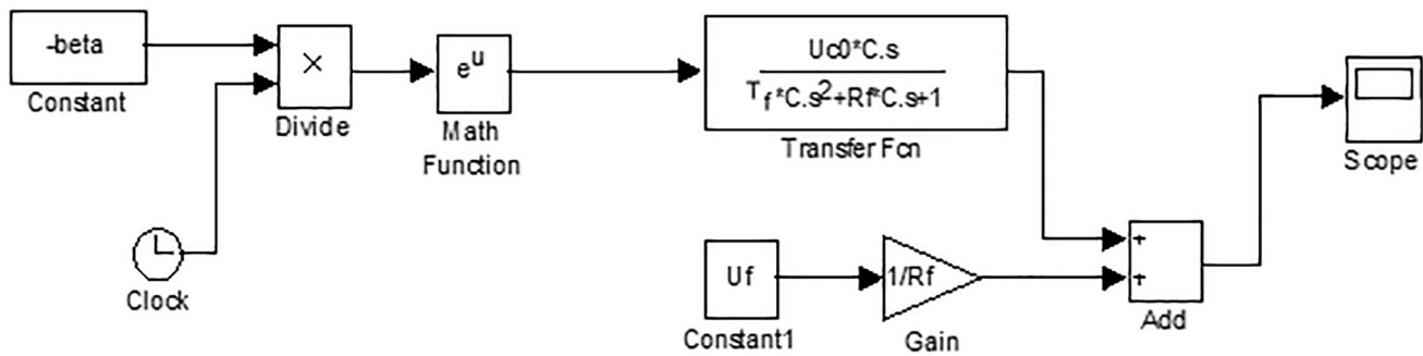
Рис. 2. Схема набору моделі компенсованого контуру збудження СГ при наявності струму збудження
