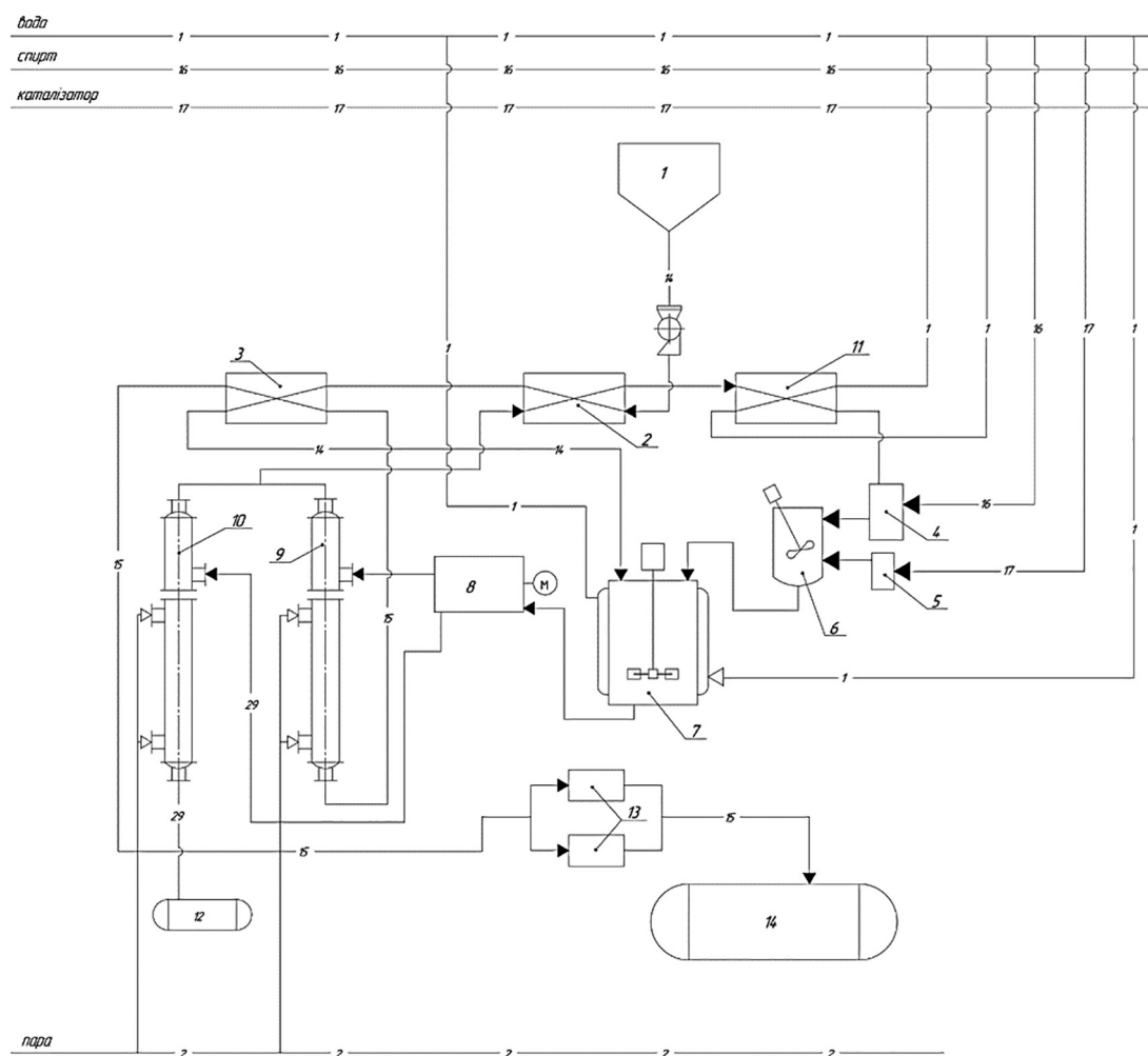
1 — ємність з олією; 2, 3 — теплообмінники; 4 — ємність з етиловим спиртом; 5 — ємність з каталізатором КОН; 6 — змішувач; 7 — реактор; 8 — центрифуга; 9, 10 — випарна колона; 11 — водяний конденсатор; 12 — збірник гліцерина; 13 — фільтри-сорбери; 14 — збірник біодизеля
