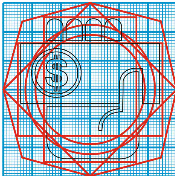
Рис. 3. Конфігуратор
