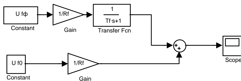
Рис. 1. Схема набору моделі некомпенсованого контуру збудження СГ
