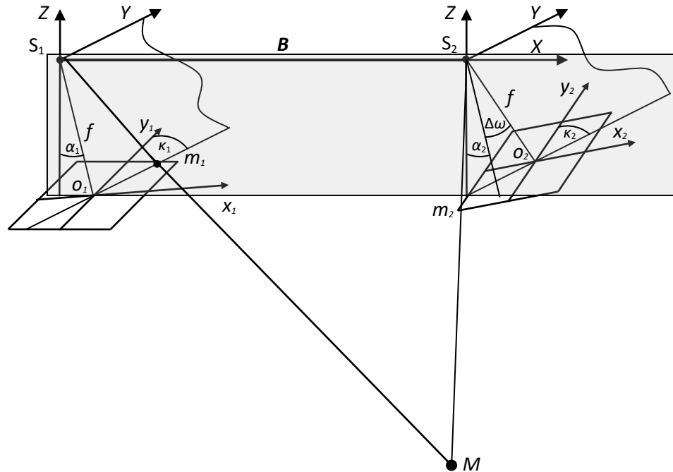
Рис. 2. Базисна система координат
