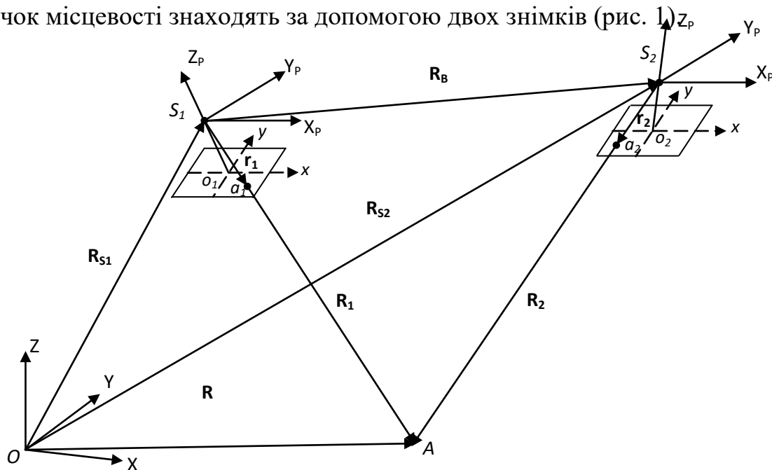
Рис. 1. Просторова фотограмметрична засічка (векторна форма запису)
