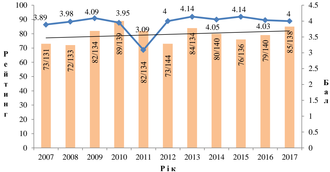
Рис. 1. Динаміка позицій та значень України в індексі глобальної конкурентоспроможності
