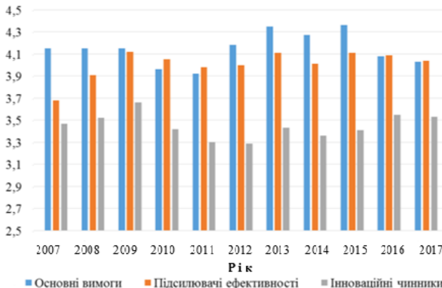
Рис. 2. Структура індексу глобальної конкурентоспроможності по секторам
