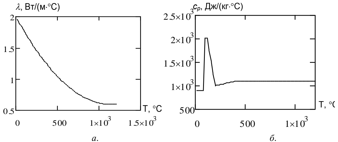
Рис. 5. Теплофізичні характеристики бетону: а – коефіцієнт теплопровідності; б – питома теплоємність
