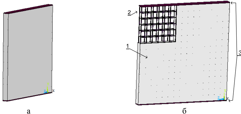
Рис. 1. Схема розрахункової області залізобетонної несучої стіни для проведення розрахунку межі вогнестійкості (а – загальний вигляд, що використовують під час обчислювального експерименту, б – схема армування): 1 –бетон, 2 –робочий арматурний каркас d = 16 мм, 3 – траверси навантажувальної рами
