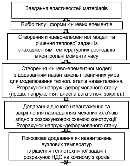
Рис. 2. Структурна схема розрахункових процедур
