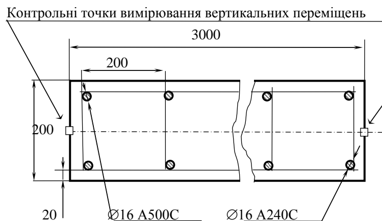
Рис. 4. Геометрична конфігурація перерізу залізобетонної стіни
