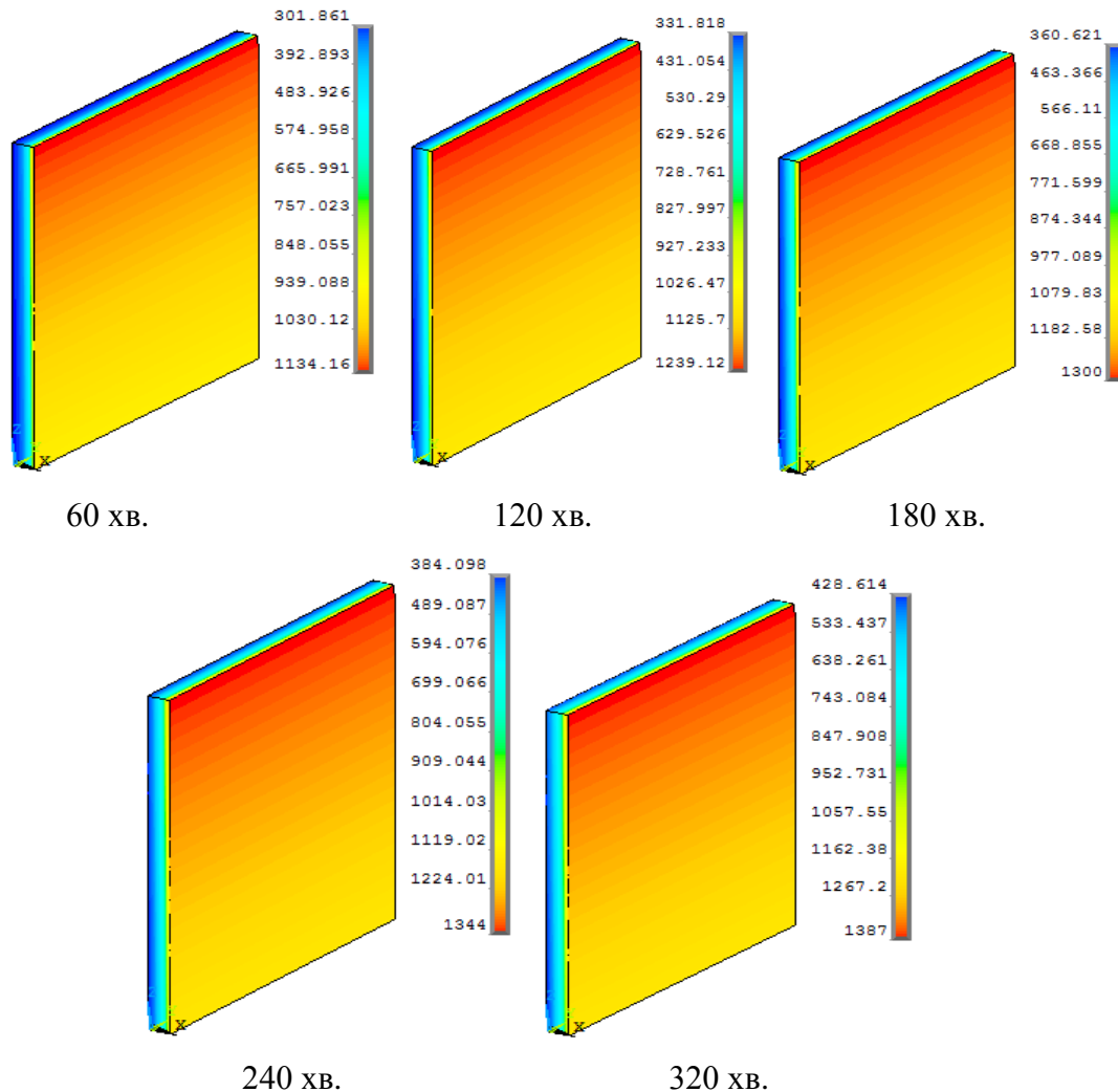
Рис. 7. Температурні розподіли (К) у залізобетонній стіні, що були отримані у результаті теплотехнічного розрахунку, у різні моменти часу її вогневого випробування
