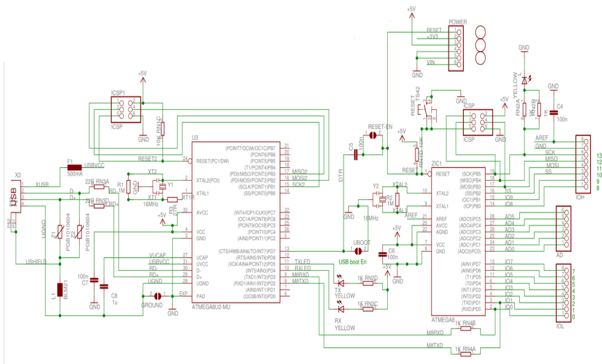
Рис. 2. Принципова електрична схема мікропроцесора Arduino Uno
