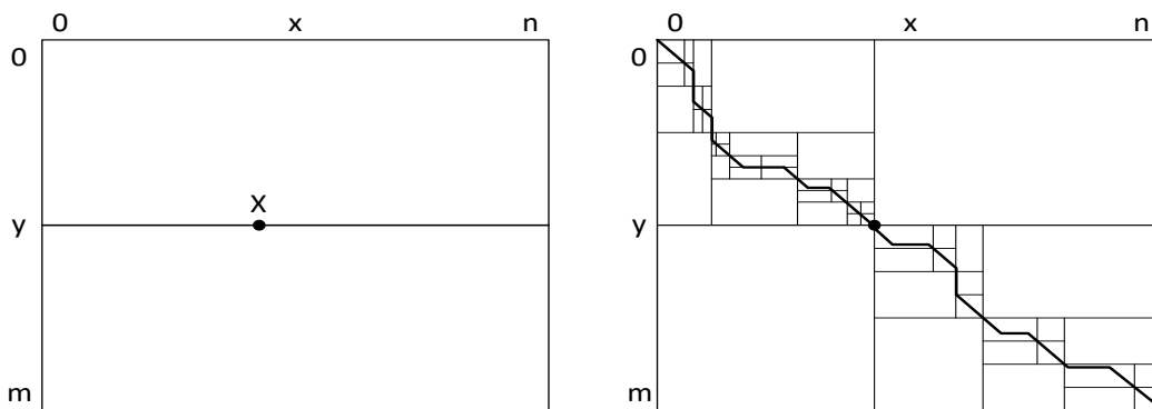
Рис. 2. Алгоритм Міллера-Маєрса
