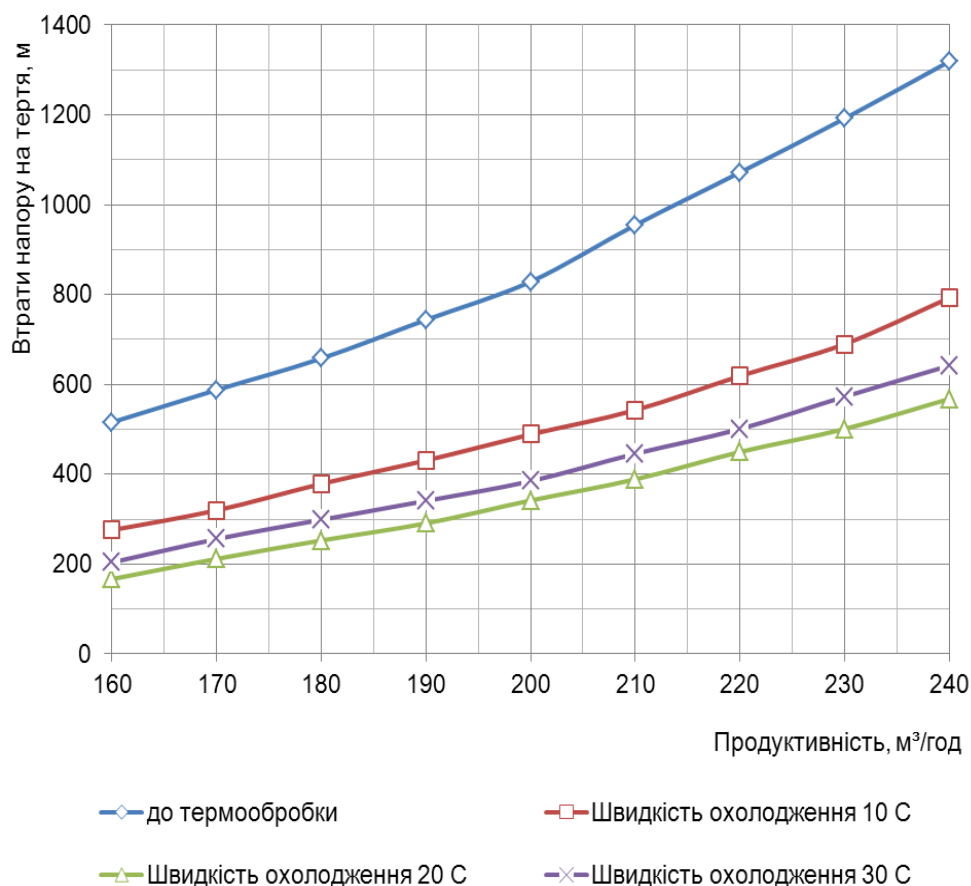
Рис. 1. Гідравлічна характеристика нафтопроводу Долина-Надвірна при перекачуванні долинської нафти до термообробки та після термообробки із різними швидкостями охолодження
