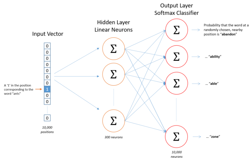
Рис. 3. Архітектура нейронної мережі моделі Word2Vec [3]
