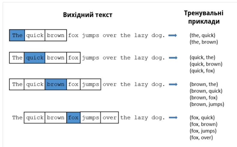
Рис. 2. Побудова тренувальних прикладів для мережі [3]
