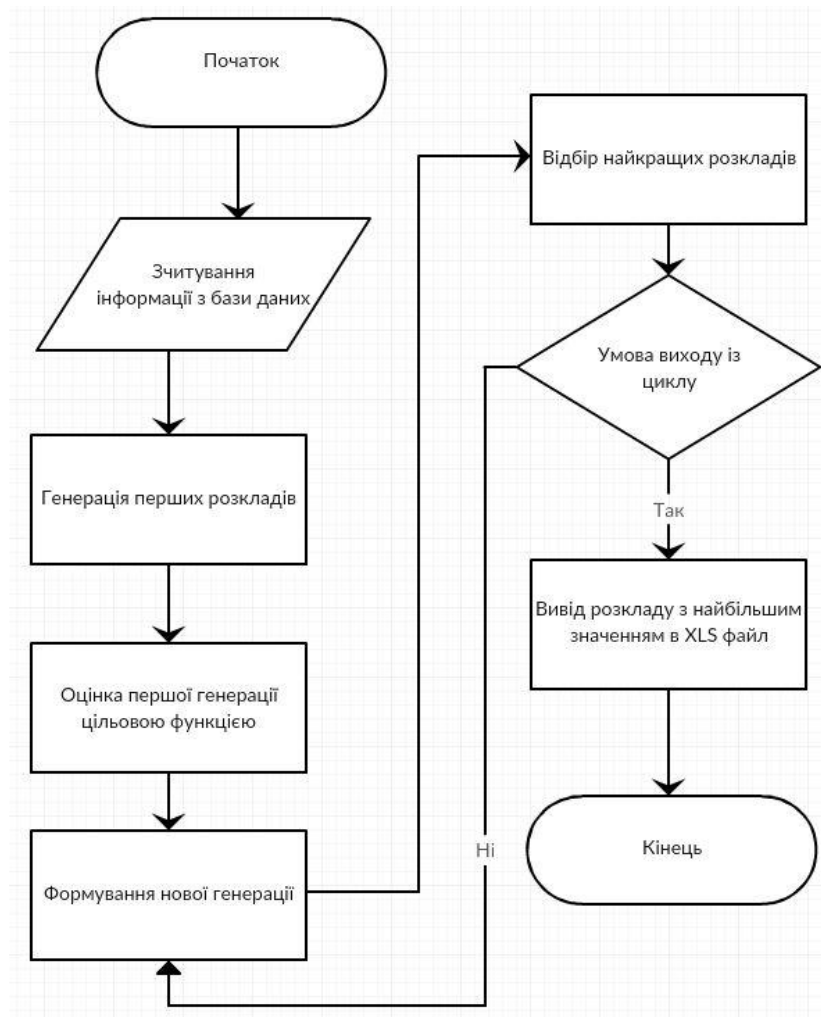
Рис. 2. Блок-схема алгоритму формування розкладу
