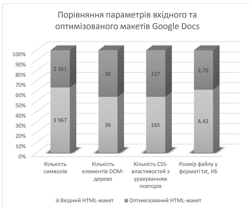
Рис. 4. Порівняння параметрів вхідного та оптимізованого макетів Google Docs
