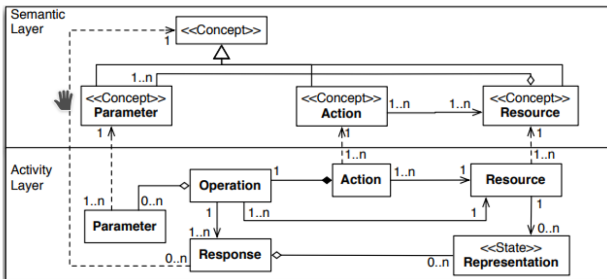
Рис. 1. Метамодель
