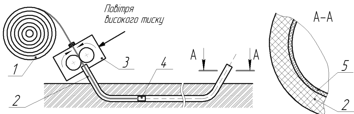
1 – бухта оптоволоконного кабелю; 2 – захисна поліетиленова труба; 3 – пристрій; 4 – парашут; 5 – антифрикційний шар
