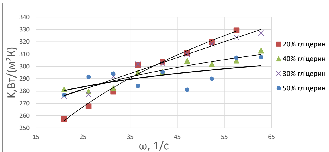
Рис. 3. Залежність коефіцієнта теплопередачі K_d від кутової швидкості для гліцерину
