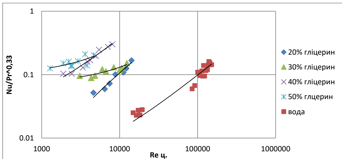
Рис. 4. Залежність \frac{Nu}{Pr^{0,33}} від критерію Рейнольдса відцентрового Re_{\text{ц}}
