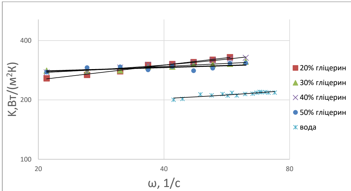
Рис. 2. Залежність коефіцієнта теплопередачі K_d від кутової швидкості для гліцерину та води
