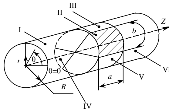
Рис. 5. Розбиття сегменту тіла на окремі об'єми
