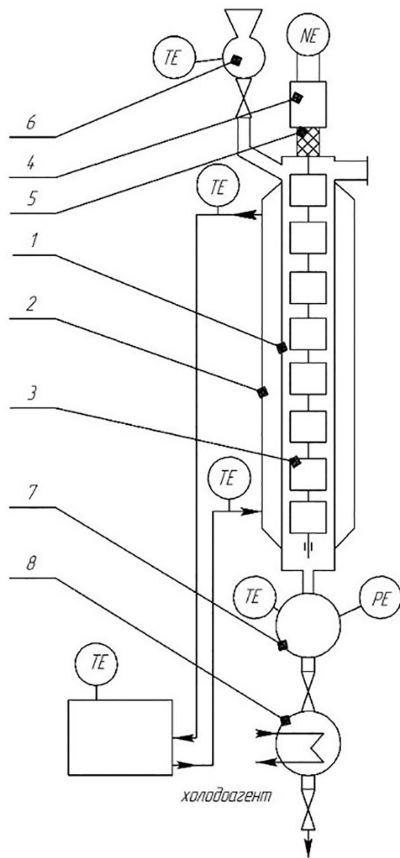
Рис. 1. Схема дослідної установки: 1 — роторний плівковий апарат; 2 — теплообмінна оболоння; 3 — шарнірний ротор; 4 — привод; 5 — ущільнення; 6 — напірний бак; 7 — приймальна ємність; 8 — зливна ємність
