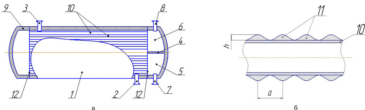
Рис. 1. Кожухотрубний теплообмінник: а) загальна схема; б) схема перерізу теплообмінної труби 1 — циліндричний кожух; 2, 3 — патрубок підведення та відведення продукту; 4 — кришка із перегородкою; 5, 6 — камера подачі та відводу теплоносія; 7, 8 — штуцери підводу та відведення; 9 — днище; 10 — теплообмінні труби; 11 — параболічні виступи; 12 — трубні решітки.
