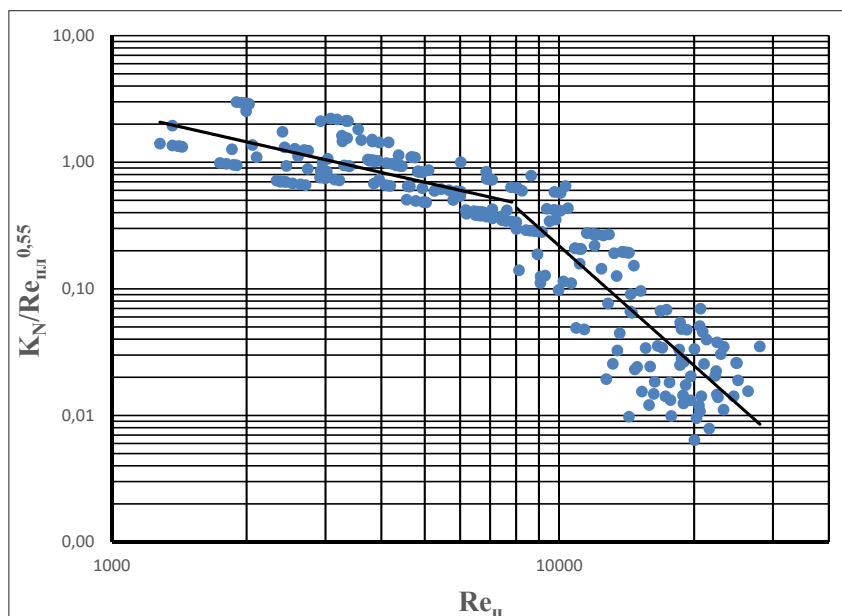
Рис. 3. Залежність коефіцієнта потужності K_N від відцентрового критерію \text{Re}_u в логарифмічній системі координат
