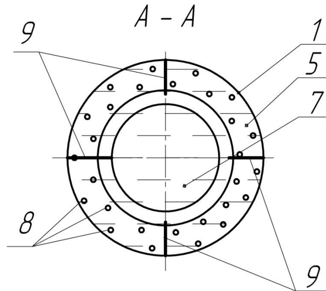
Рис. 2. Переріз А-А на рис. 1 газліфтного барботажного апарату
