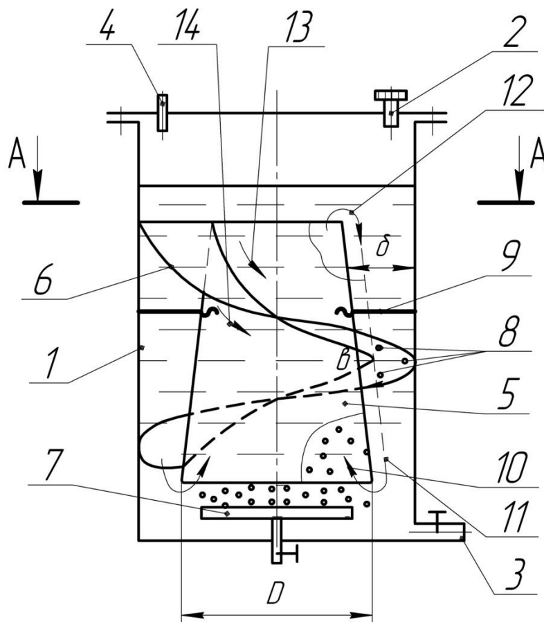
Рис. 1. Газліфтний барботаажний апарат
