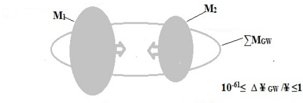
Рис. 1. Схема регистрации гравитационно-волновой амплитуды массы GW от слияния двух массивных черных дыр и формула эволюции новообразованной массы
