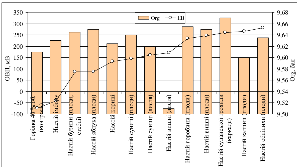
Рис. 3. Графічна залежність органолептичних показників та енергії відновлення рослинних водно-спиротових настоїв
