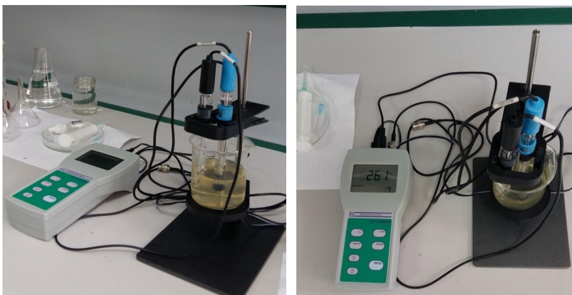
Рис. 2. Експериментальне дослідження водно-спиртових настоїв за фізико-хімічними показниками: рівнем рН та ОВП
