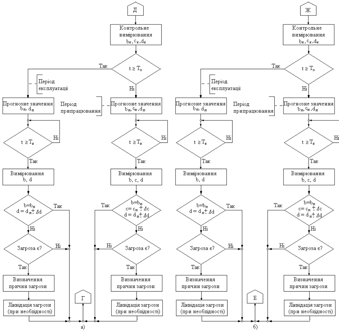
Рис. 3. Алгоритм організації вимірювальних робіт в процесі експлуатації будівель і споруд (середня та висока уразливість)
