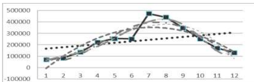
Рис.1. Оптимальный выбор математической модели для общих объемов реализации продукции: а- 2003г. (в литрах); б - 2013г.(в тыс. драмах РА). —■— - исходные данные, ...- прямая регрессионная связь, - - -, — · —, - - -, · - ·, соответственно степенные функции 2-6-го порядков
