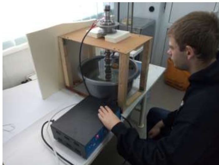
Рис. 3. Ультразвуковий випромінювач в дії
