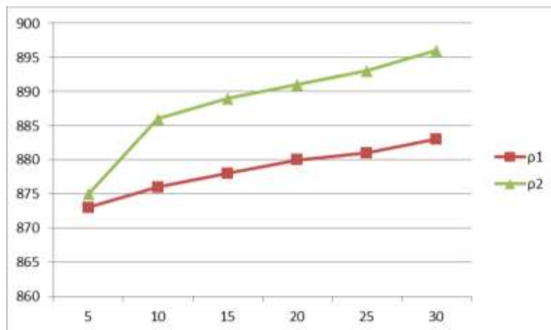
Рис. 2. Графік залежності густини від часу \rho_{c1} -без ультразвуку, \rho_{c2} - з ультразвуком
