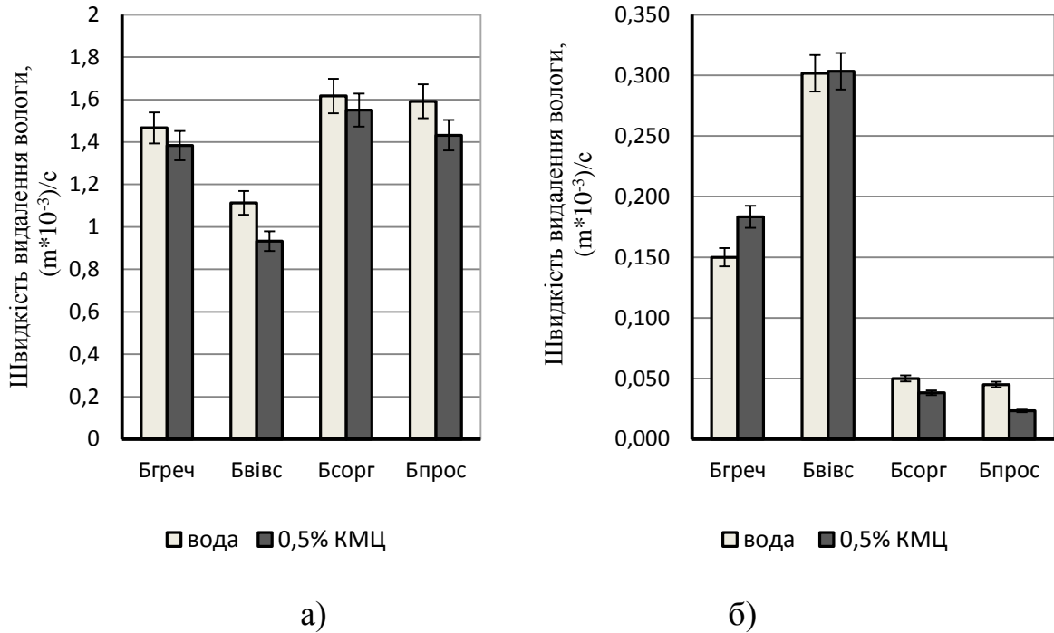
Рис. 3. Швидкість видалення вологи зі зразків тіста з різного видів борошна:
