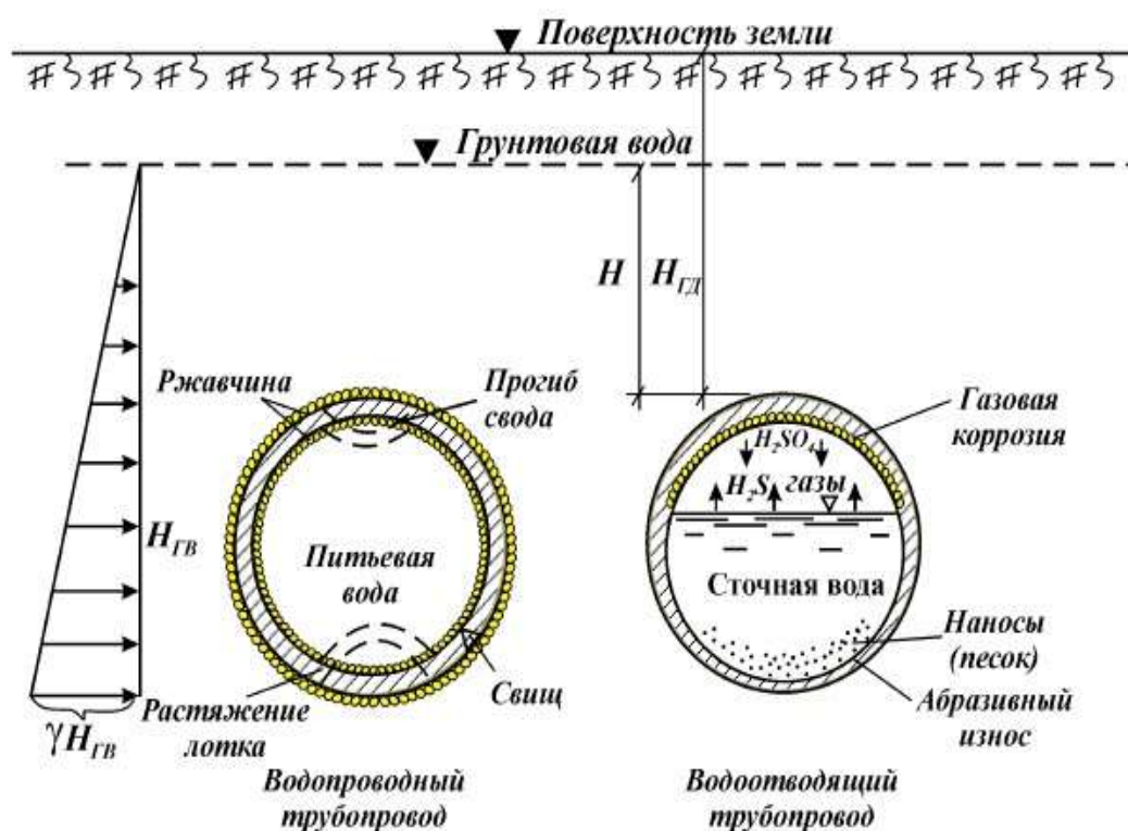
Рис. 1. Иллюстрация воздействия на трубопроводы нагрузок, приводящих к нарушению режима работы
